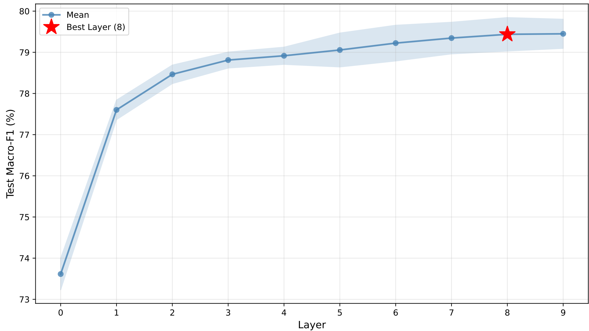
Adult - Test Macro-F1
