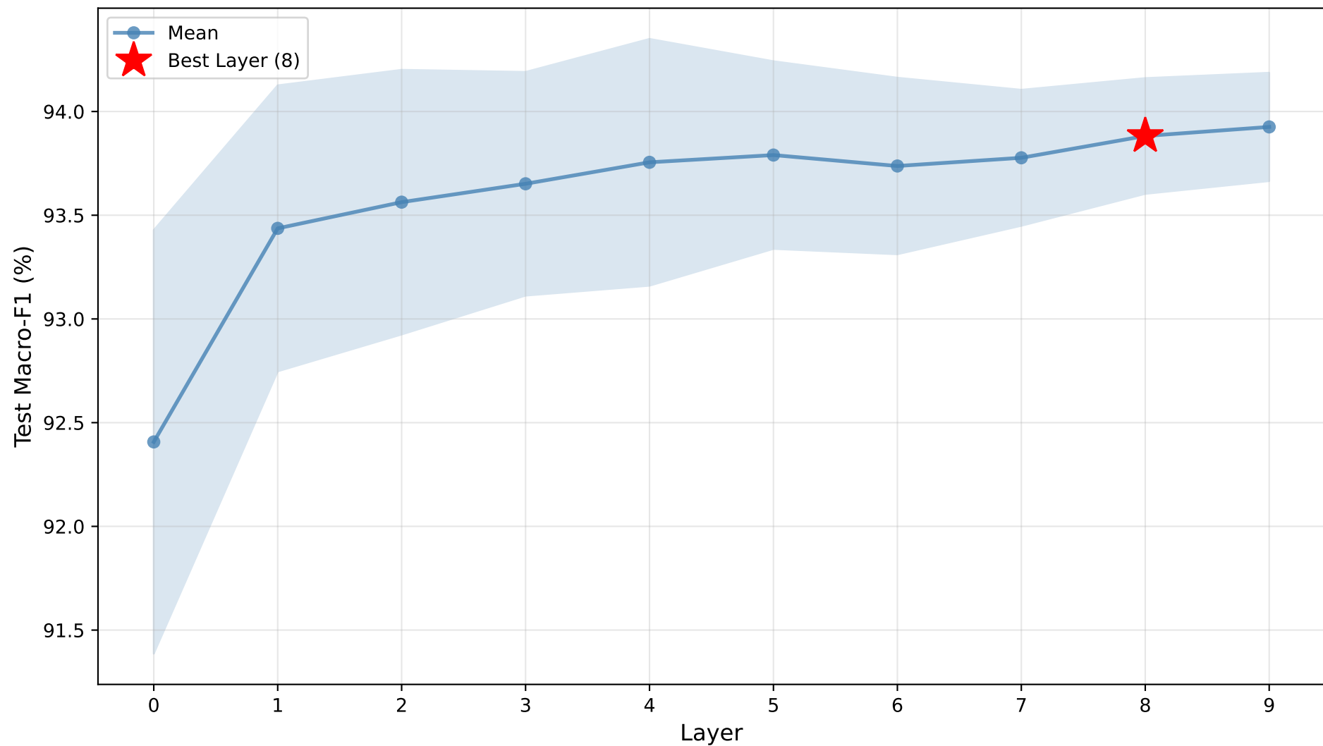
DNA - Test Macro-F1
