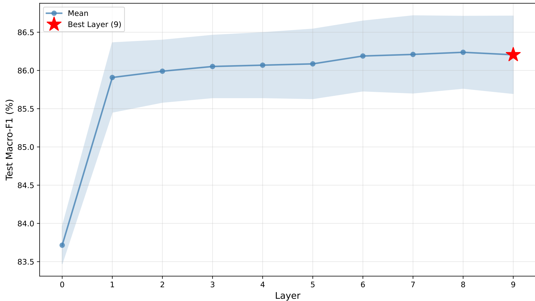
Gamma - Test Macro-F1
