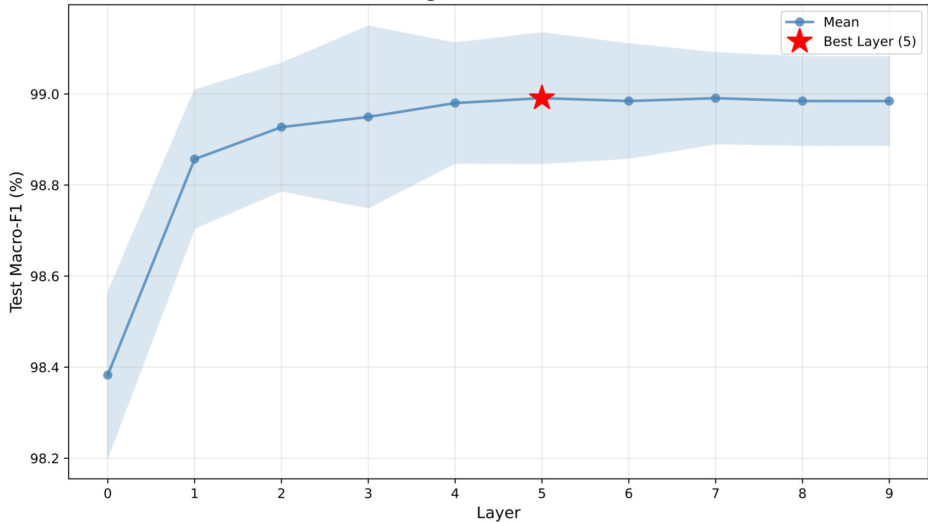
Pendigits - Test Macro-F1
