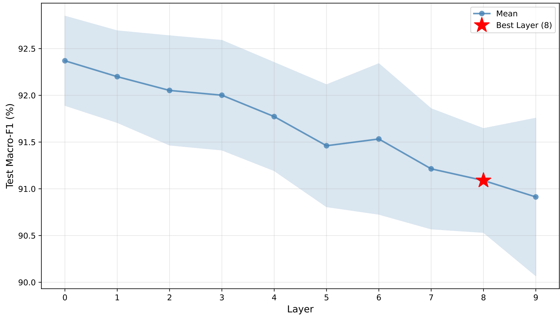
Rice - Test Macro-F1
