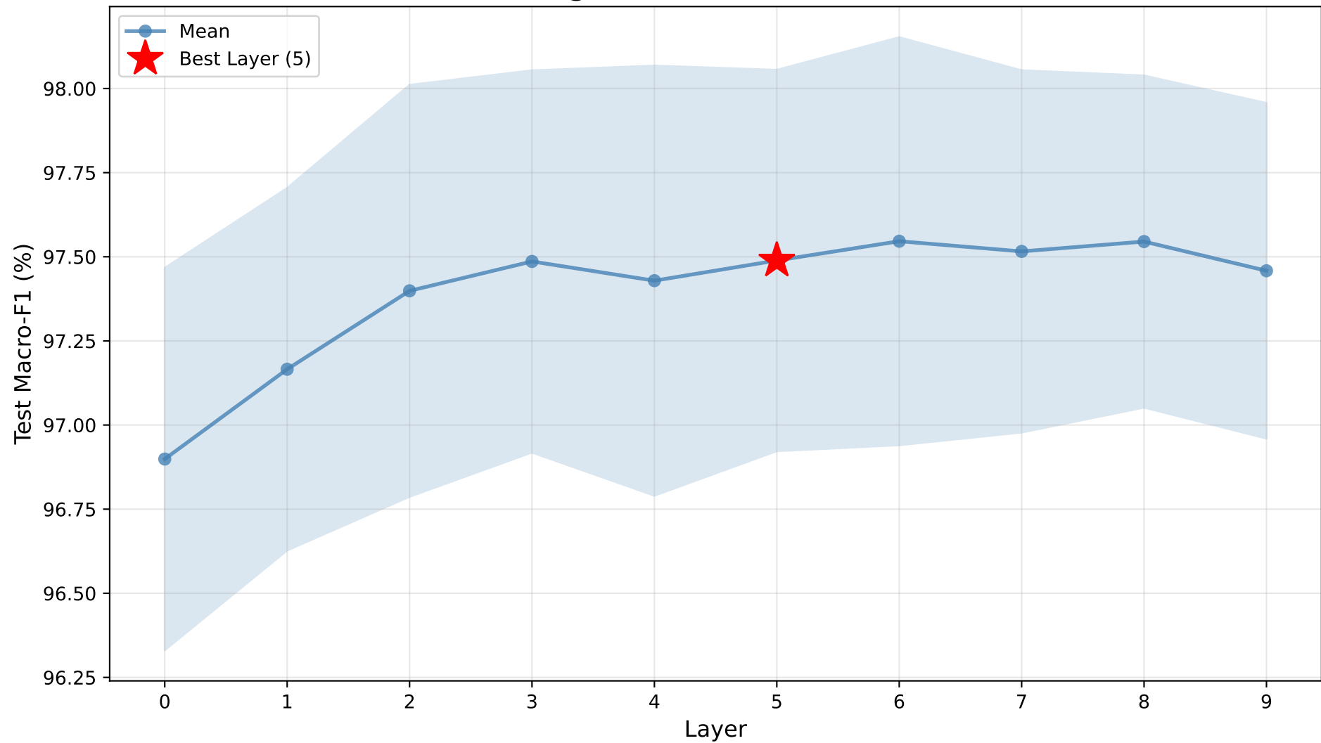
Segment - Test Macro-F1
