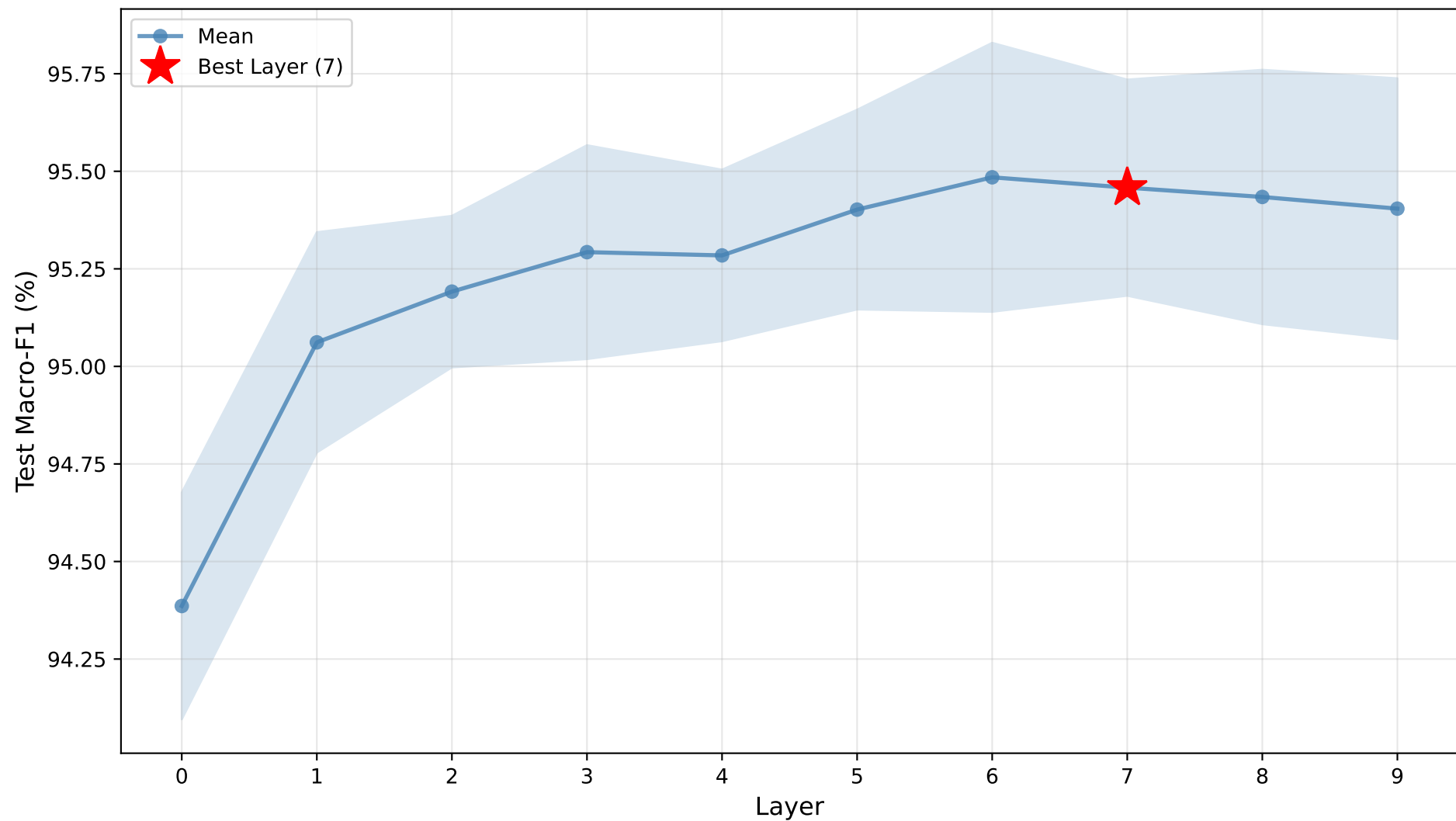
USPS - Test Macro-F1
