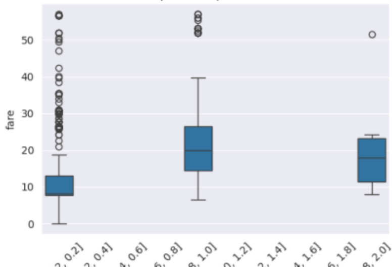
fare / sibsp (Découpés en intervalles)
