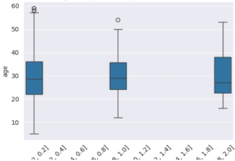
age / sibsp (Découpés en intervalles)
