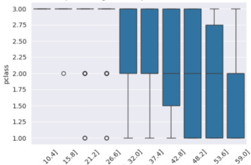
pclass / age (Découpés en intervalles)
