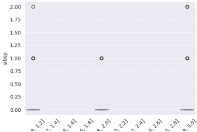
sibsp / pclass (Découpés en intervalles)
