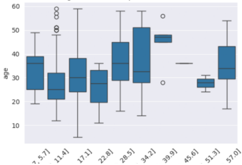
age / fare (Découpés en intervalles)
