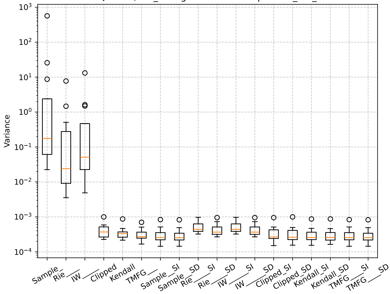
Q=1.60, len_rolling=100: Box Plot per min_var_
