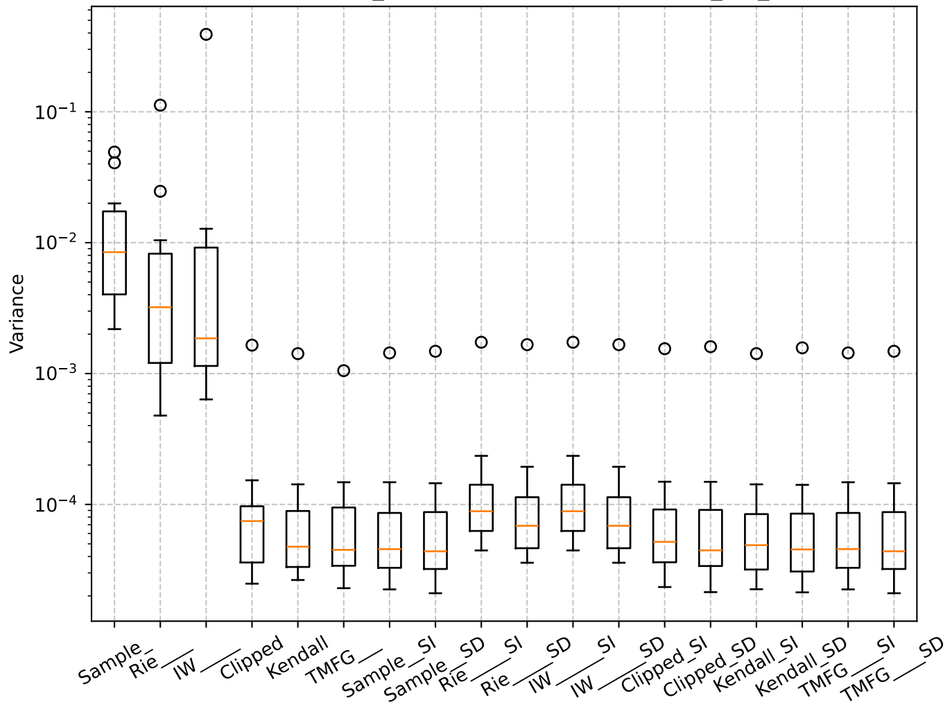
Q=3.33, len_rolling=100: Box Plot per min_var_
