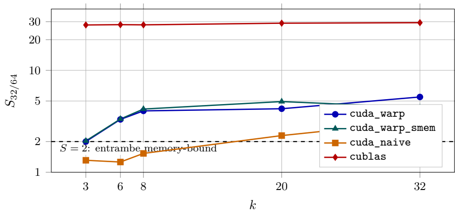
Figura 7.8: Fase 3: guadagno della singola precisione al variare di k . La crescita con k dei kernel custom è la previsione del roofline, la piatezza di cublas intorno a 28 misura invece la lentezza del suo percorso FP64.
