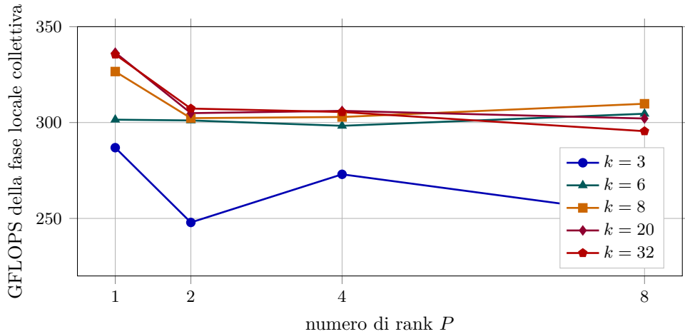
Figura 7.9: Fase 4: throughput collettivo di cuda_warp a S = 16384 per la famiglia di griglie della tabella 7.16.
