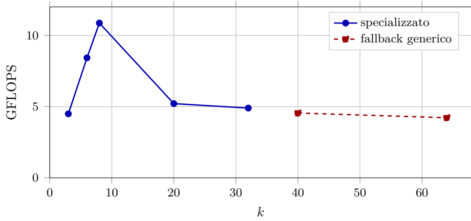
Figura 6.1: C3: prestazioni del nucleo di CPU al variare di k . Il massimo cade a k = 8 ; oltre, il throughput crolla.
