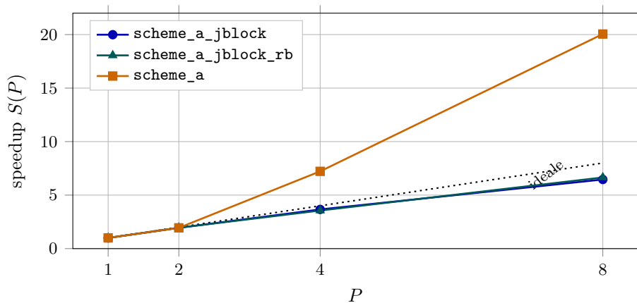
Figura 7.11: Analisi CPU a S = 16384 e k = 32 : speedup sulla migliore griglia per ogni P . La crescita superlineare di scheme_a misura un cambio di regime della cache, non un aumento sovrilineare delle risorse.
