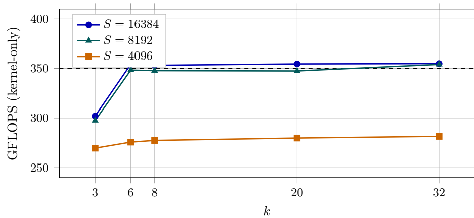
Figura 7.8: Fase 2: cuda_warp sul caso quadrato alle tre scale. La linea tratteggiata è il tetto FP64 nominale. A S = 4096 la curva non arriva al tetto per nessun k .
