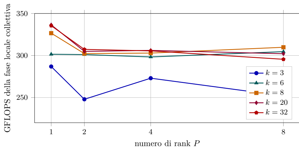
Figura 7.10: Fase 4: throughput collettivo di cuda_warp a S = 16384 per la famiglia di griglie della tabella 7.15.
