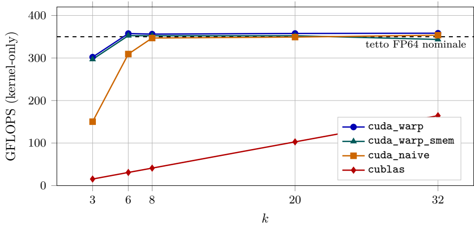
Figura 7.7: Confronto fra i backend configurati sul problema di riferimento in doppia precisione. La linea tratteggiata rappresenta il tetto FP64 nominale utilizzato nel modello roofline.
