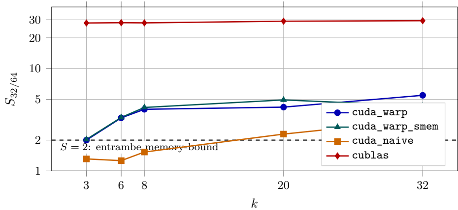
Figura 7.9: Fase 3: guadagno della singola precisione al variare di k . La crescita con k dei kernel custom è la previsione del roofline, la piatezza di cublas intorno a 28 misura invece la lentezza del suo percorso FP64.
