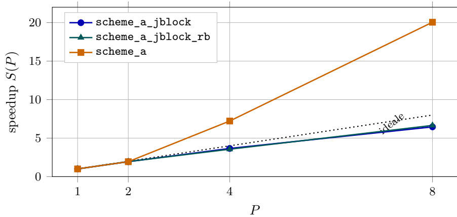
Figura 7.11: Analisi CPU a S = 16384 e k = 32 : speedup sulla migliore griglia per ogni P . La crescita superlineare di scheme_a misura un cambio di regime della cache, non un aumento sovralineare delle risorse.
