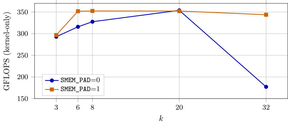
Figura 7.4: Campagna 1.3: confronto fra tile senza padding e con una colonna di padding. Il caso k = 32 rende visibile la patologia che negli altri punti è parzialmente nascosta dal resto del lavoro del kernel.
