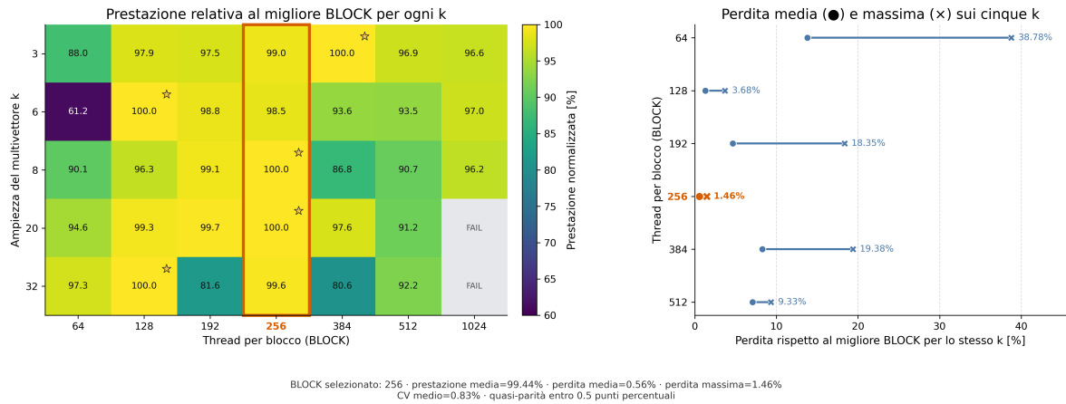
(b) cuda_warp_smem.
