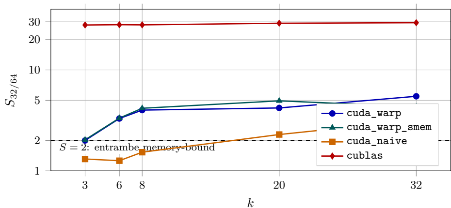
Figura 7.9: Fase 3: guadagno della singola precisione al variare di k . La crescita con k dei kernel custom è la previsione del roofline, la piatezza di cublas intorno a 28 misura invece la lentezza del suo percorso FP64.
