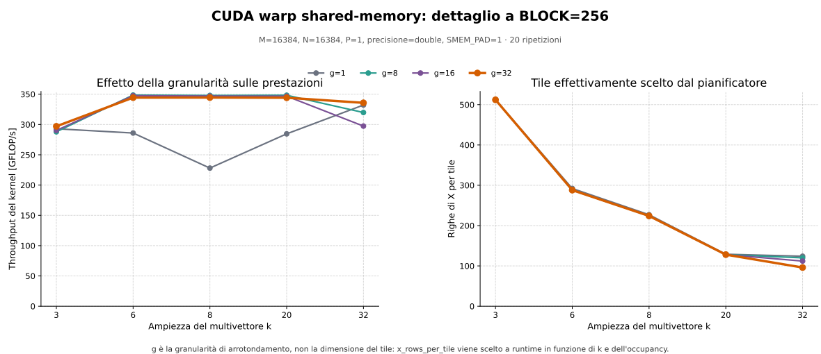
Figura 7.6: Campagna 1.4: dettaglio a BLOCK= 256. A destra il piano di tiling effettivamente scelto a runtime, che dipende da k e non da g se non attraverso l'arrotondamento.
