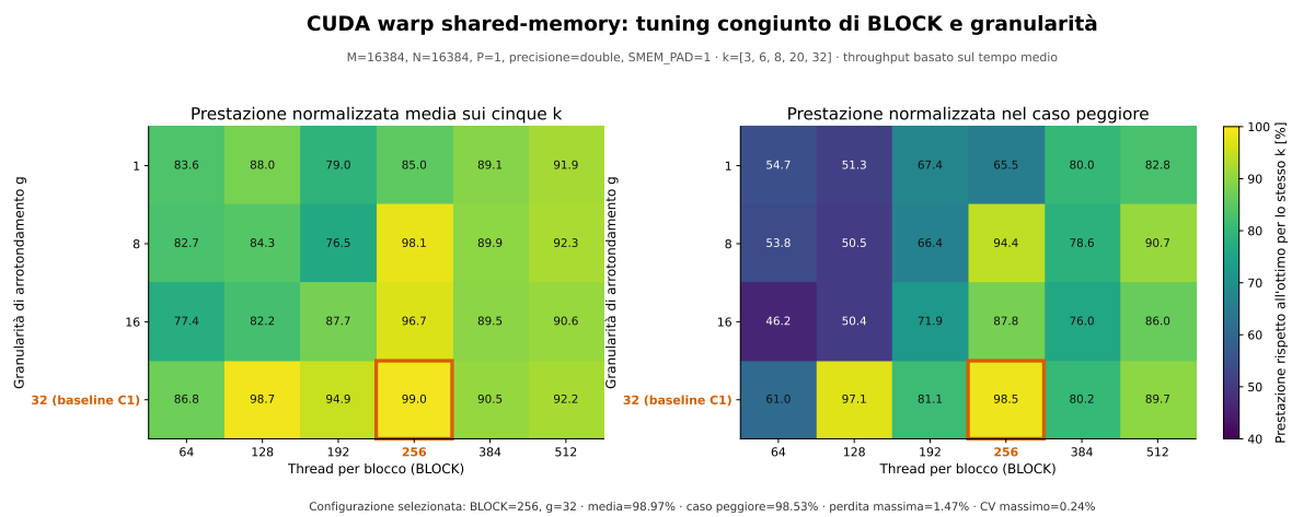
Figura 7.5: Campagna 1.4: tuning congiunto di BLOCK e granularità. A sinistra la prestazione normalizzata media sui cinque k , a destra il caso peggiore.
