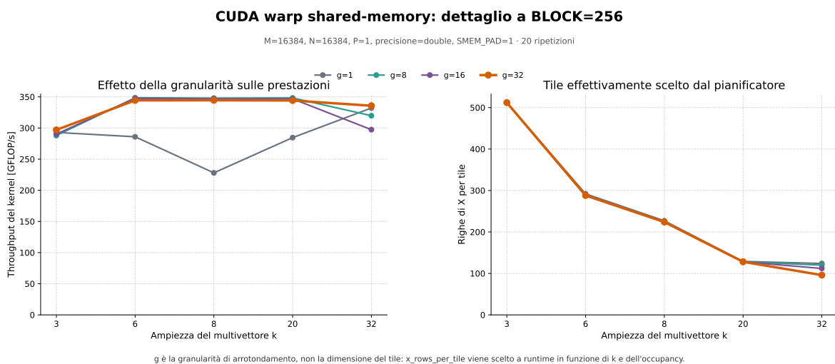
Figura 6.5: Campagna 1.3: dettaglio a BLOCK= 256. A destra il piano di tiling effettivamente scelto a runtime, che dipende da k e non da g se non attraverso l'arrotondamento.
