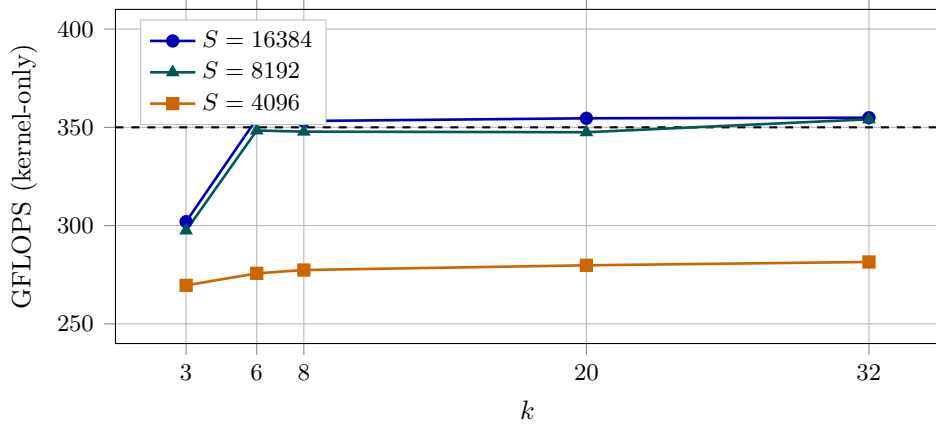
Figura 6.7: Fase 2: cuda_warp sul caso quadrato alle tre scale, dai valori della tabella 6.7. La linea tratteggiata indica il tetto FP64 nominale di 350 GFLOP/s utilizzato nel modello.
