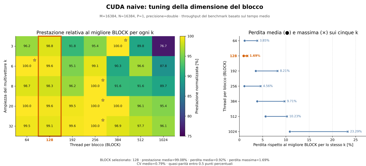
Figura 6.2: Campagna 1.1: stessa lettura per cuda_naive, l'unico kernel che completa anche a BLOCK= 1024.
