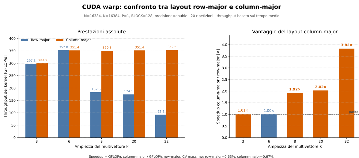
Figura 6.3: Campagna 1.2: prestazioni assolute (sinistra) e vantaggio del layout column-major (destra). CV massimo: 0,63% row-major, 0,67% column-major.
