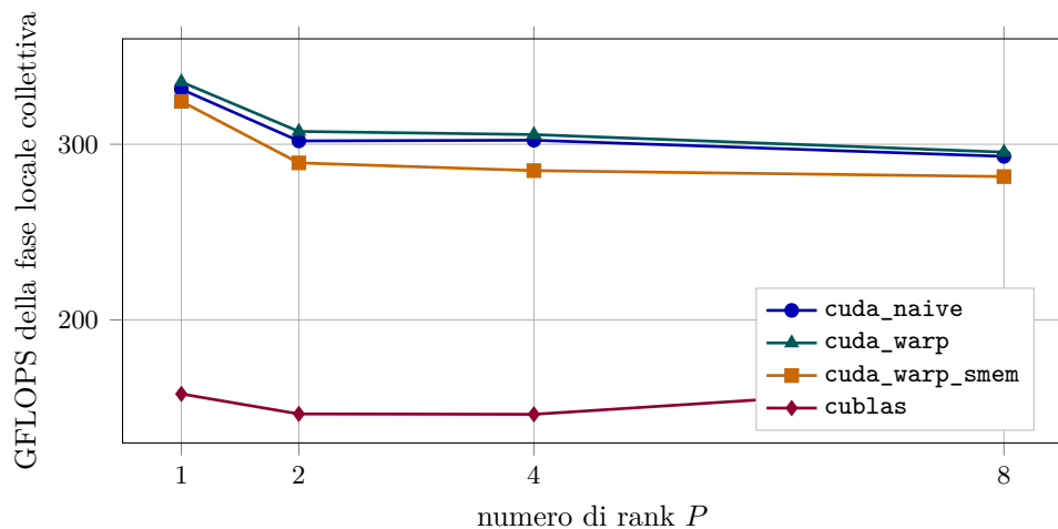
Figura 6.8: Fase 4: throughput collettivo a S = 16384 e k = 32 per i quattro backend, dalla colonna corrispondente della tabella 6.15.
