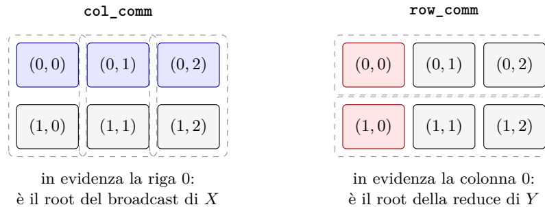
Figura 3.2: La stessa griglia, raggrupata nei due modi. Fissando la coordinata di riga si ottengono i comunicatori row_comm , fissando quella di colonna i comunicatori col_comm . Ogni processo appartiene a esattamente uno di ciascun tipo, e i due si intersecano soltanto in lui.
