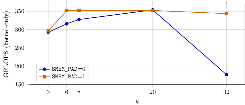
Figura 6.6: Campagna 1.4: confronto fra tile senza padding e con una colonna di padding. Il caso k = 32 rende visibile la patologia che negli altri punti è parzialmente nascosta dal resto del lavoro del kernel.
