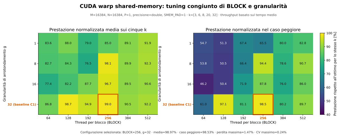
Figura 6.4: Campagna 1.3: tuning congiunto di BLOCK e granularità. A sinistra la prestazione normalizzata media sui cinque k , a destra il caso peggiore.
