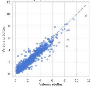
Ridge : prédictions vs réalité
