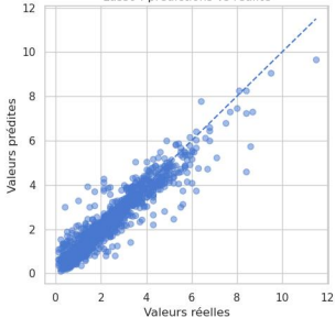
Lasso : prédictions vs réalité
