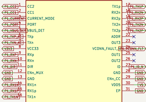
U600 HD3SS3220IRNHR
