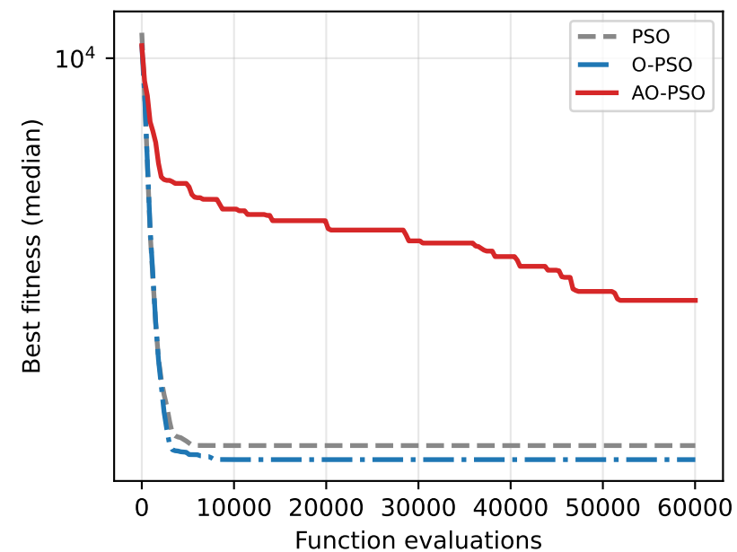
Schwefel
