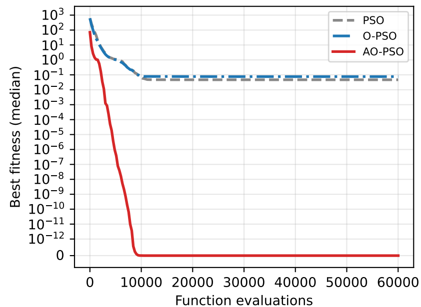
Griewank
