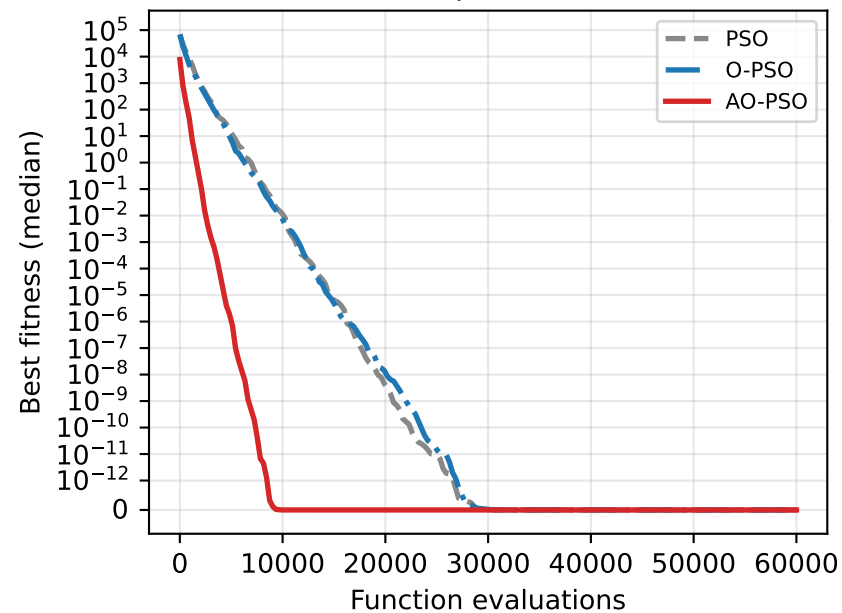
Griewank
