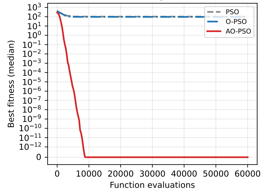
Schwefel
