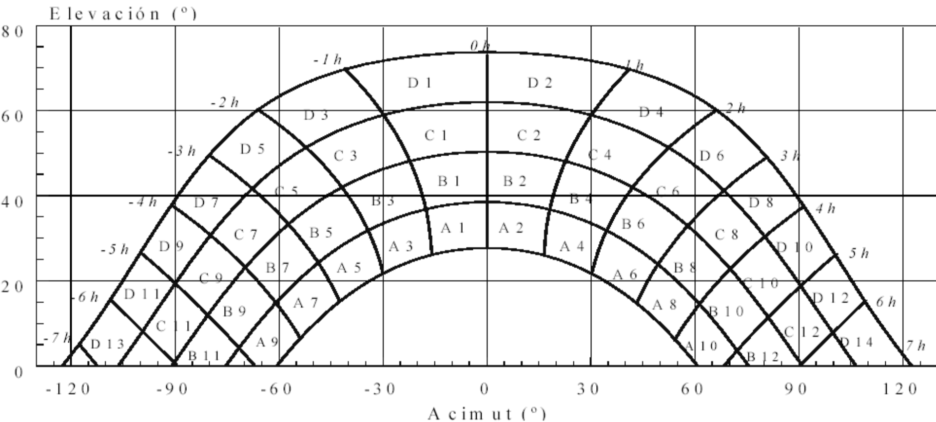
Figura 3.4 Diagrama de trayectorias del sol
