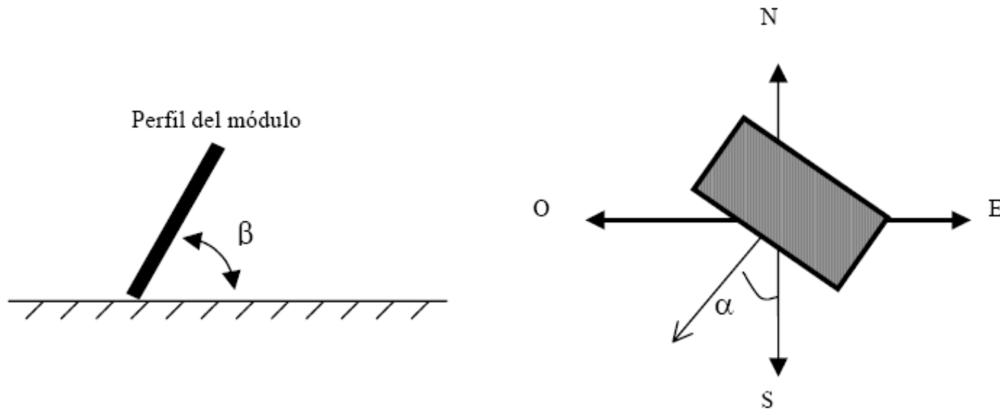
Figura 3.2 Orientación e inclinación de los módulos
