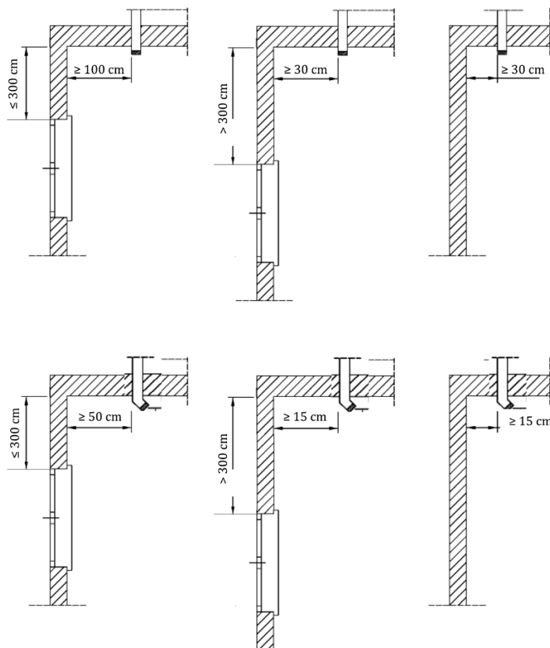
Figura 13 – Distancias a guardar por el conducto de evacuación de los productos de la combustión respecto a paredes laterales
