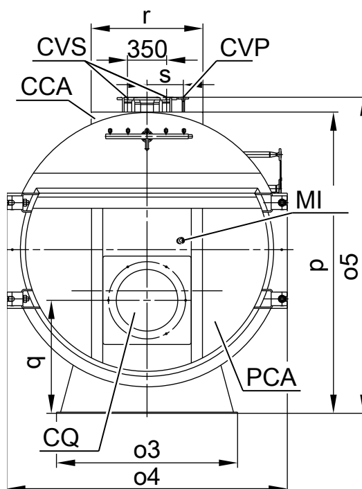
Figura 2.3. Esquema de la caldera Viessmann VITOMAX 100-HS M33A (sin economizador). Fuente: Catálogo Viessmann. Elaboración grupal.
