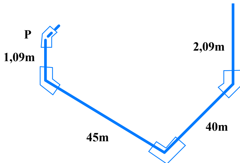
Figura A.9. Esquema del Tramo 2 de Condensados (P-C1). Fuente: Elaboración grupal.
