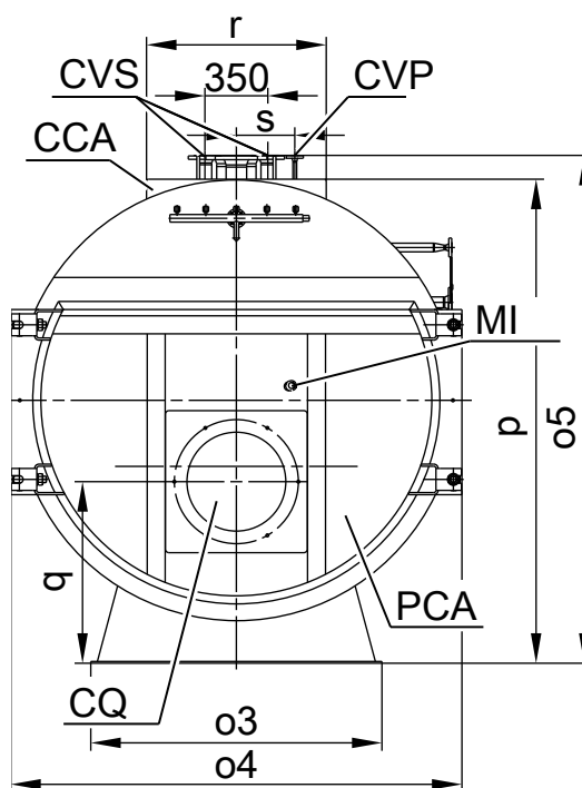
Figura 2.3. Esquema de la caldera Viessmann VITOMAX 100-HS M33A (sin economizador). Fuente: Adaptada de [1].
