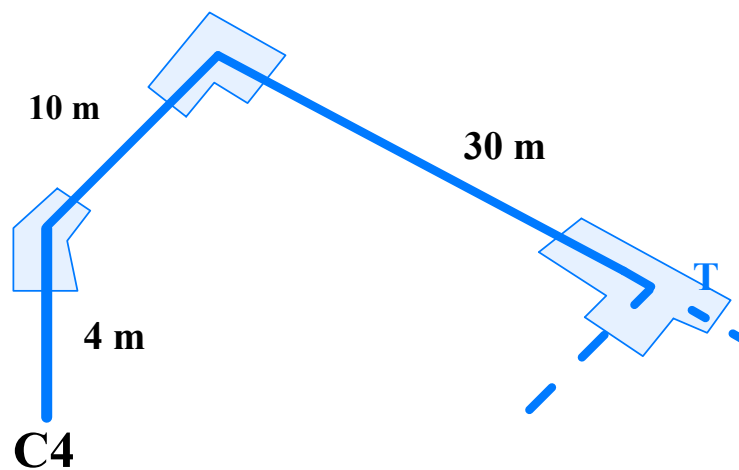
Figura A.14. Esquema del Tramo 7 de Condensados (T-C4). Fuente: Elaboración grupal.
