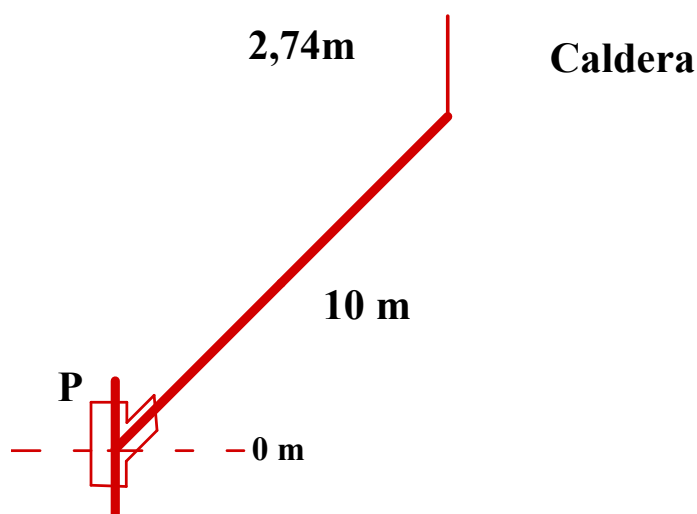
Figura 2.6. Croquis del Tramo 1 (Caldera-P). Fuente: Elaboración grupal. Nota: Este diagrama también se incluye en la Figura A.1 del Anexo 2 para referencia detallada.
