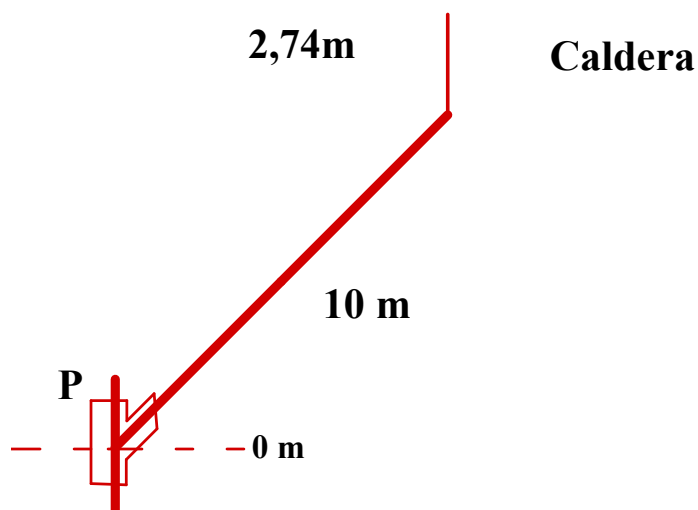
Figura A.1. Esquema del Tramo 1 de Vapor (Caldera-P). Fuente: Elaboración grupal.
