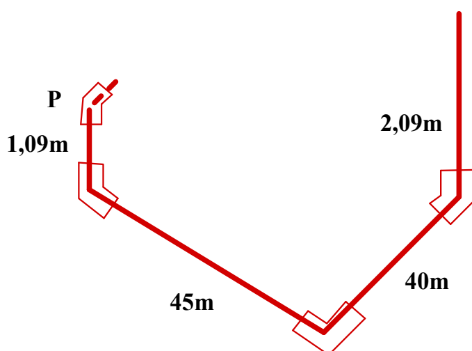
Figura A.2. Esquema del Tramo 2 de Vapor (P-C1). Fuente: Elaboración grupal.
