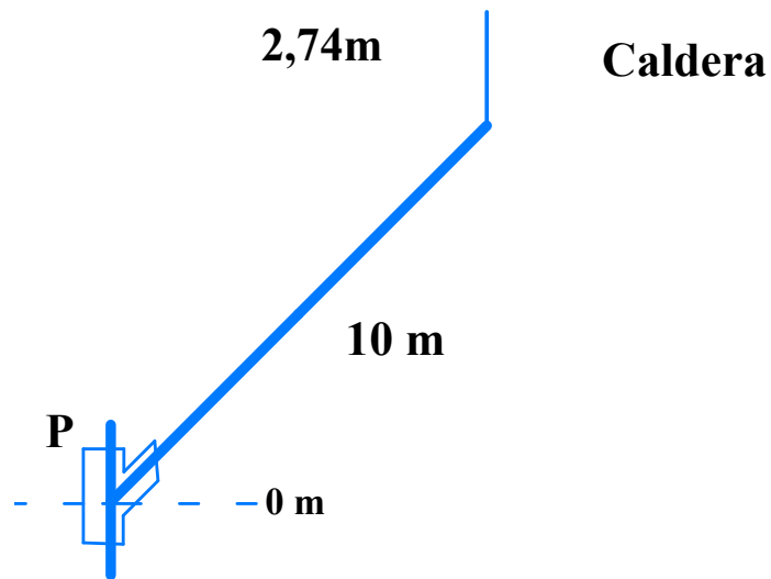
Figura A.8. Esquema del Tramo 1 de Condensados (Caldera-P). Fuente: Elaboración grupal.
