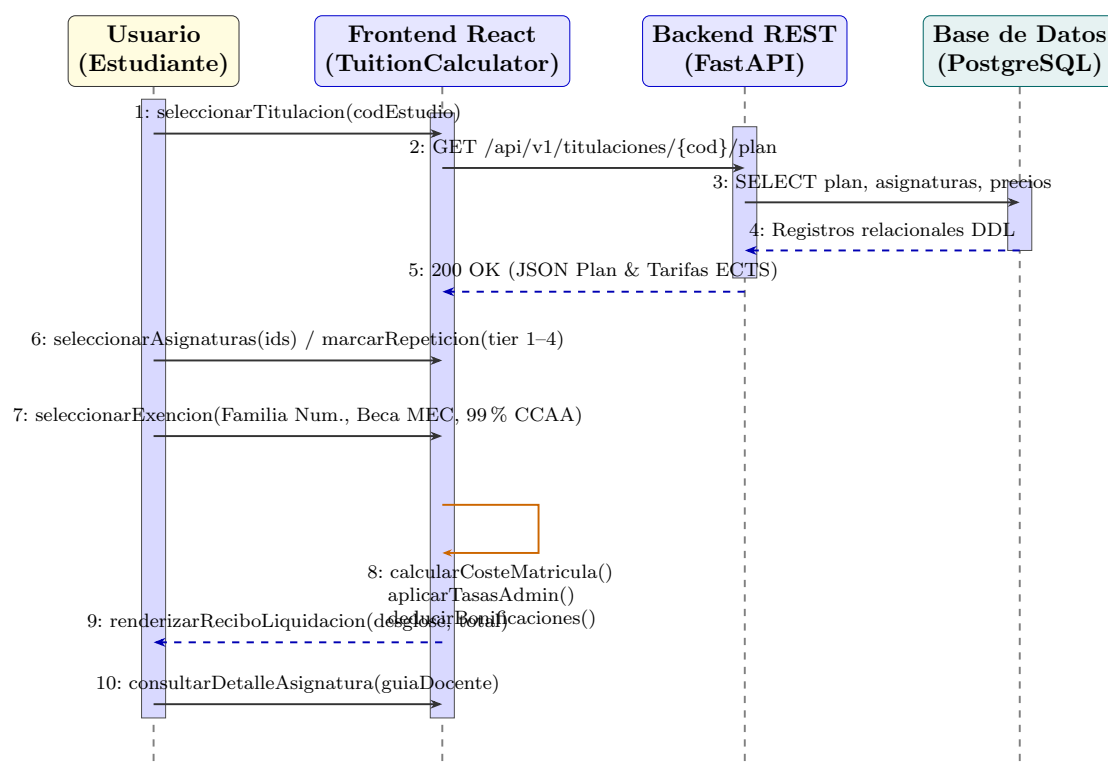
Figura 5.4: Diagrama de Secuencia UML: Interacción en la Simulación Financiera de Matrícula (Fase 3)
