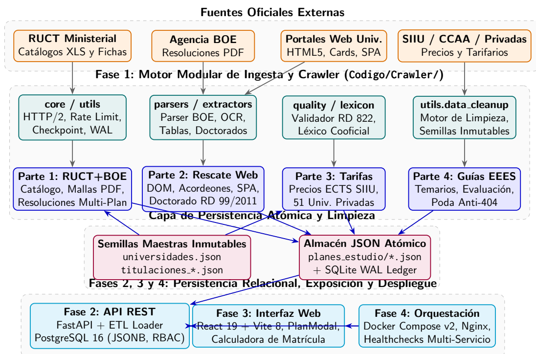
Figura 7.1: Estructura modular y flujo interno de procesamiento de datos en UniHub.
