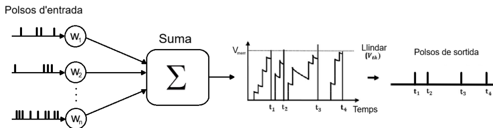
Figura 15: Evolució temporal del potencial de membrana V(t) en una neurona LIF, mostrant l'efecte de la fuga i la generació de spikes. Font: [30]
