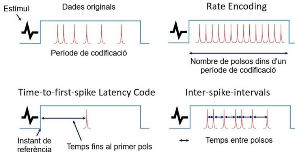
Figura 16: Comparació entre codificació per taxa i codificacions temporals. Font: [31]
