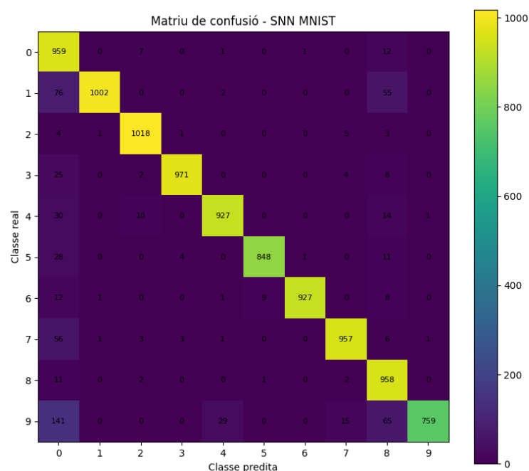
Figura 22: Matriu de confusió del model SNN per la classificació de dígitos manuscrits.
