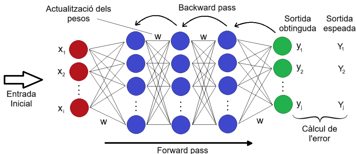
Figura 6: Flux de dades i actualització de pesos en la retropropagació.
