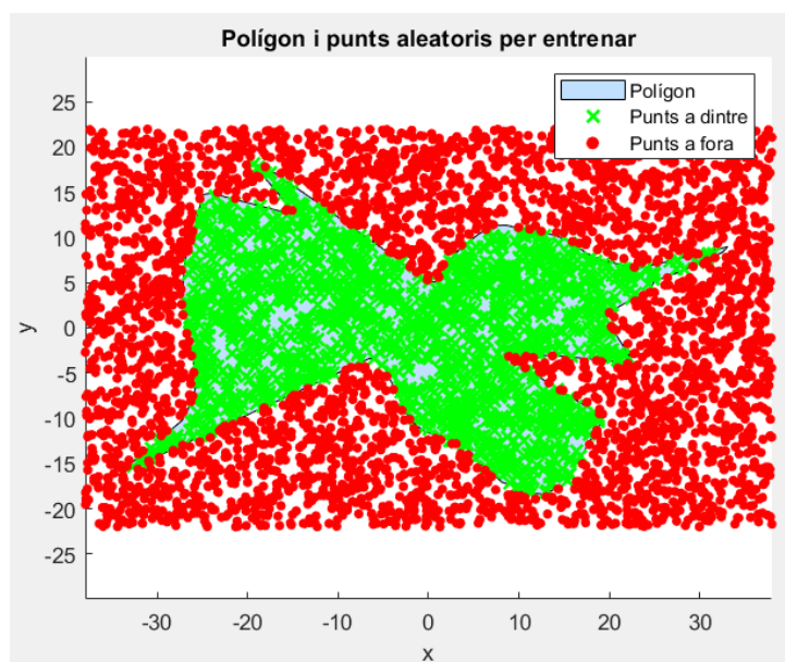
Figura 18: Dades d'entrenament generades, amb punts de classe 0 (fora del polígon) en vermell i punts de classe 1 (dins del polígon) en verd.
