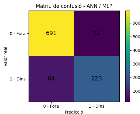
Figura 19: Matriu de confusió del model ANN per la classificació de punts.
