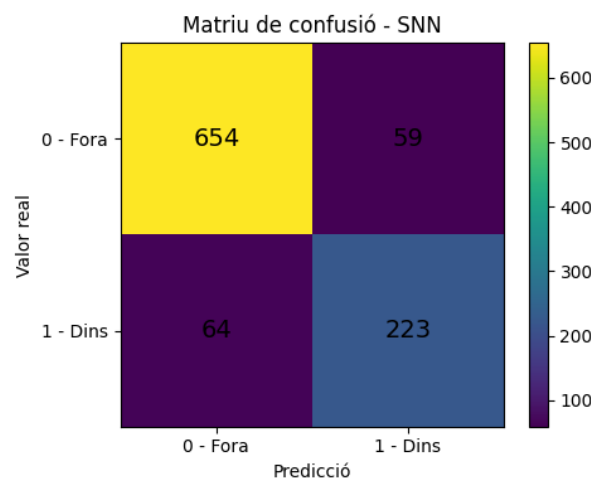
Figura 20: Matriu de confusió del model SNN per la classificació de punts.
