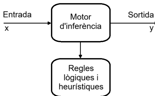
Figura 2: Il·lustració del funcionament de la Good Old-Fashioned AI (GOFAI).
