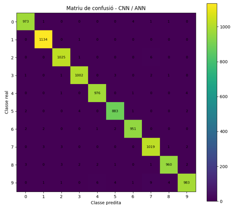
Figura 21: Matriu de confusió del model CNN per la classificació de dígitos manuscrits.
