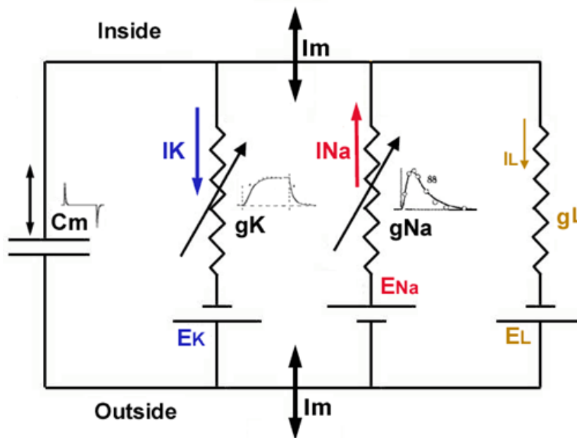
Figura 10: Circuit equivalent del model de Hodgkin-Huxley amb canals iònics dependents del voltatge. Font: [27]
