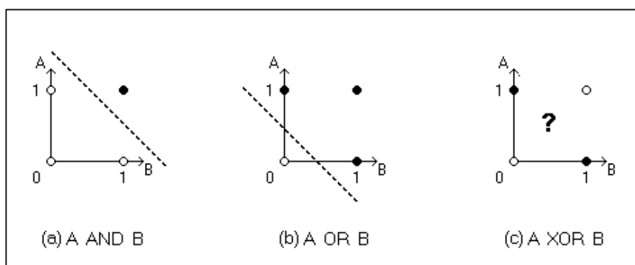
Figura 4: Problemes linealment separables i no linealment separables. Font: [12].
