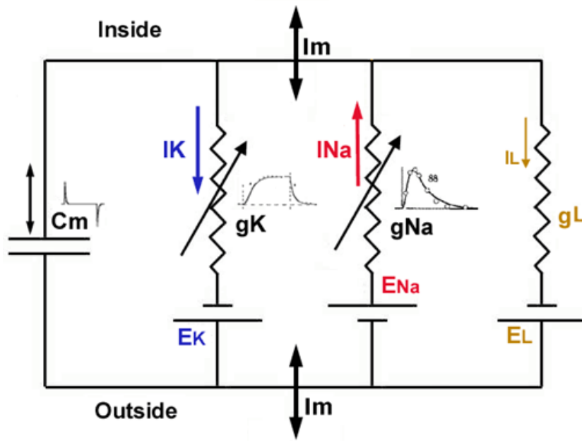
Figura 11: Circuit equivalent del model de Hodgkin–Huxley amb canals iònics dependents del voltatge. Font: [27]
