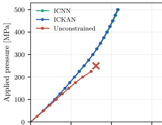
(d) Compression in x
