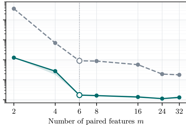
(b) ICKAN core
