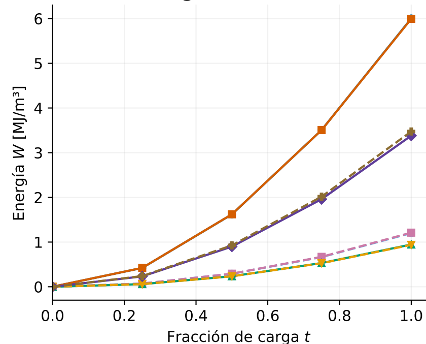
(c) Energía de deformación
