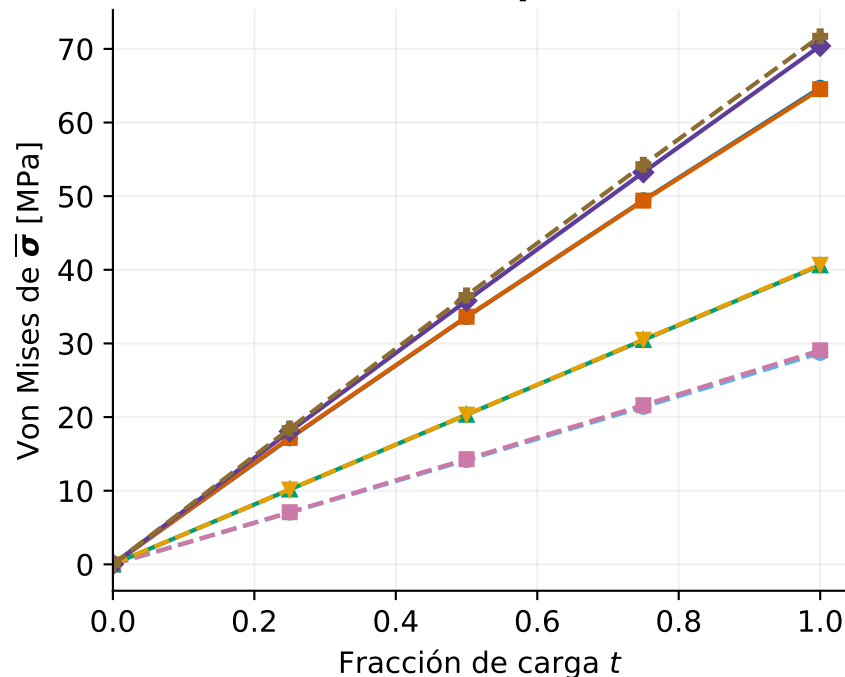
(b) Tensión equivalente
