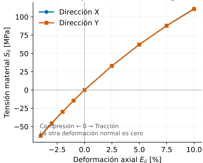
(a) Respuesta axial con signo
