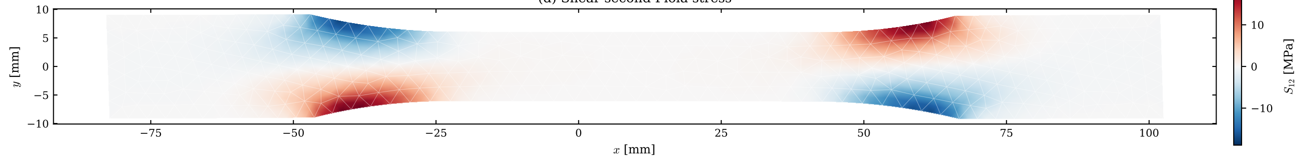
(d) Shear second Piola stress
