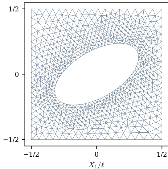
Periodic cell: 1546 T6 elements
