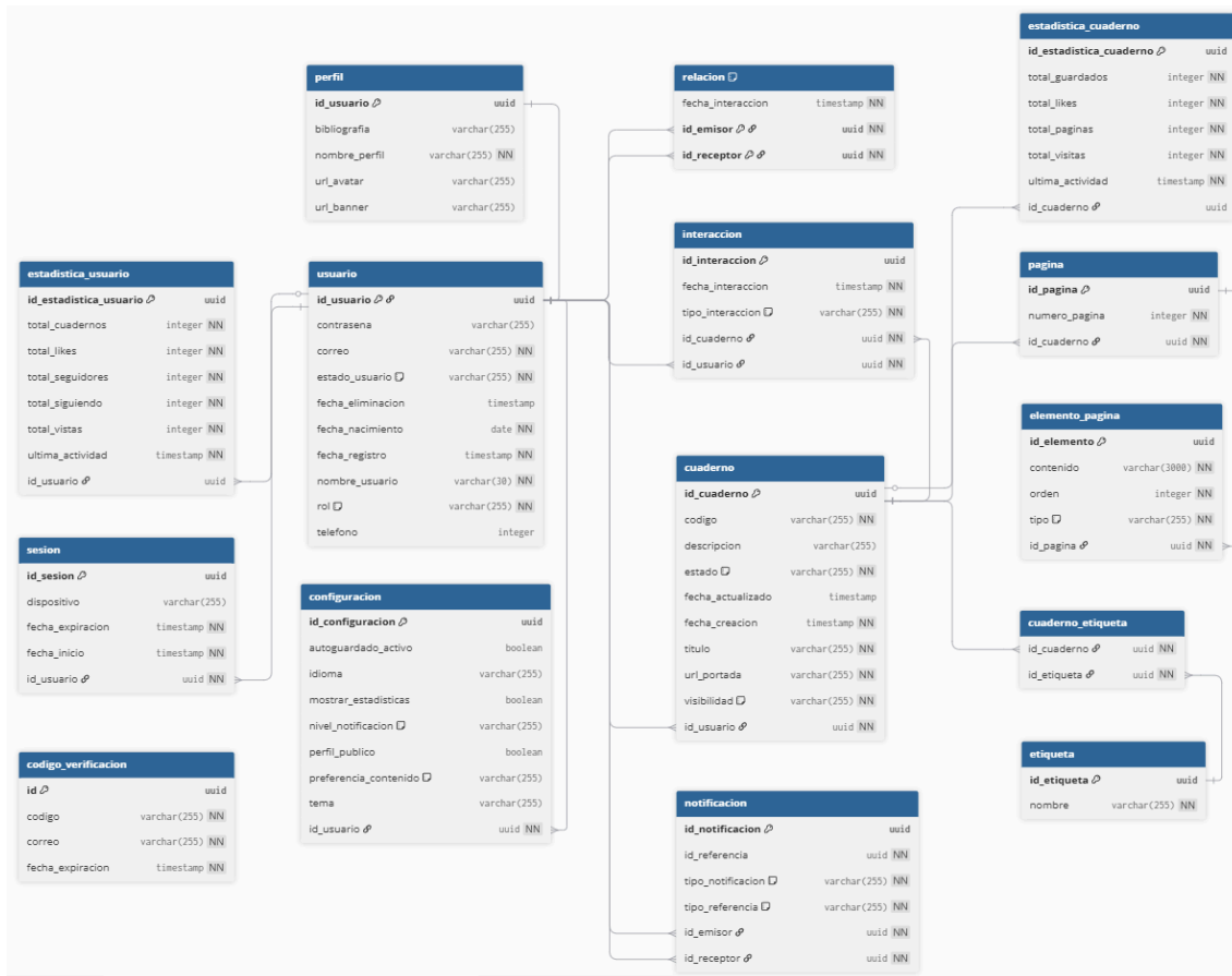
Ilustración 14 : Mapa de Base de Datos. Fuente: dbdiagram.io
