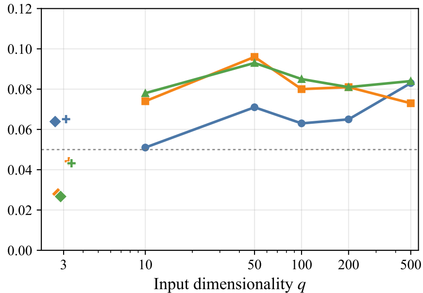
(d) Sparse PCA, Task f_E : phase transfer
