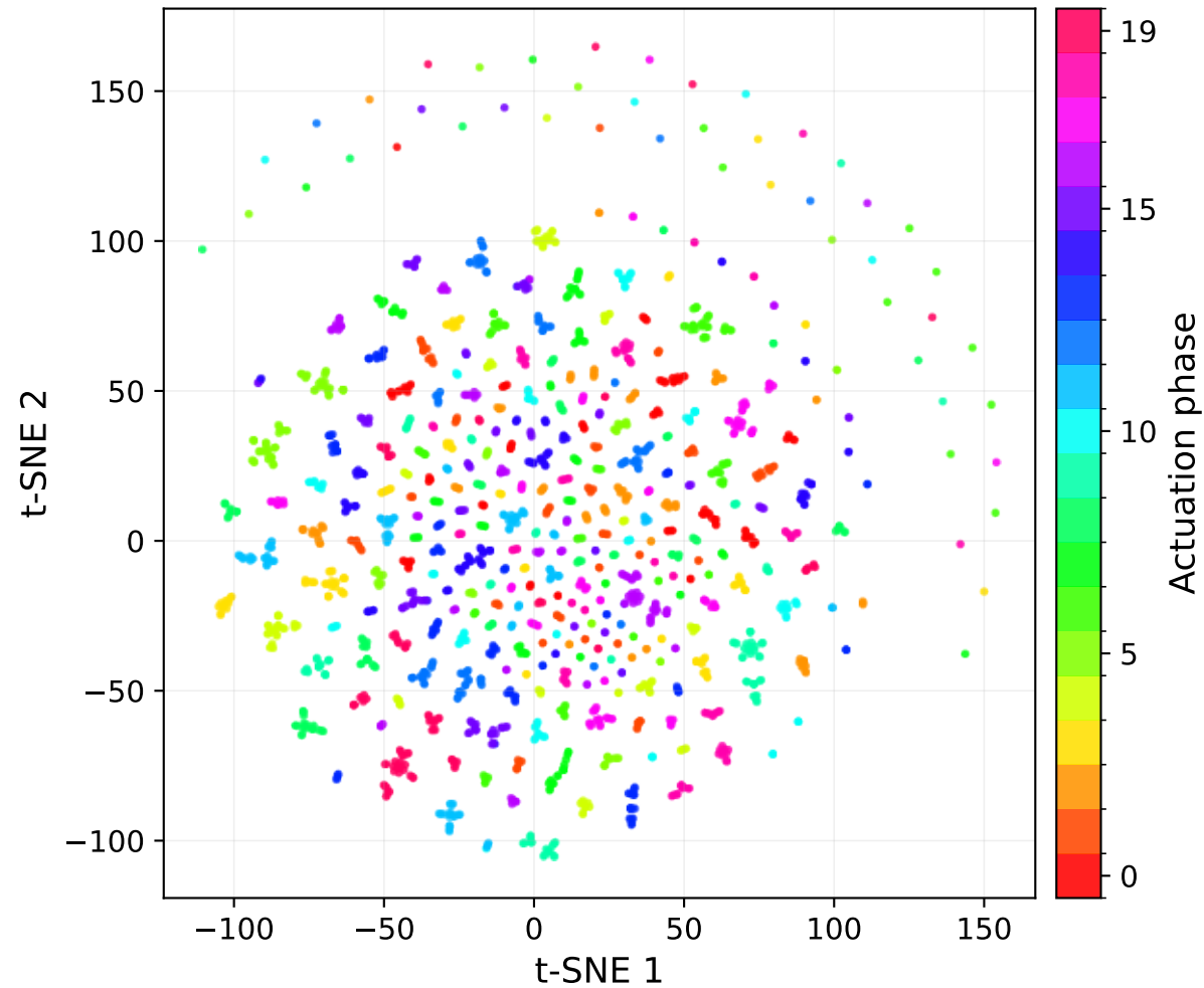
RUN2 original-space t-SNE, St_{act} = 0.05
