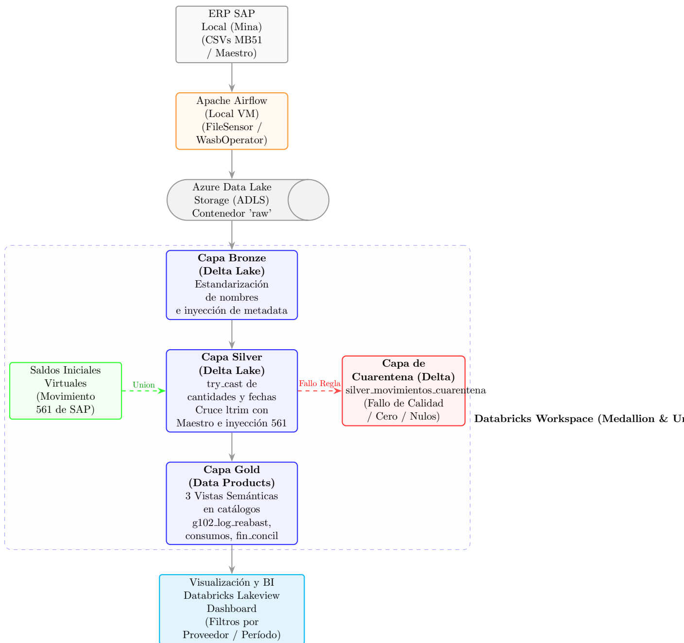
Figura 1: Flujo técnico y arquitectura de datos detallada de inventarios.
