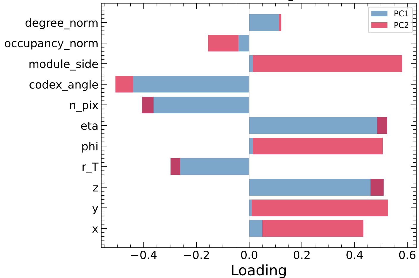
PCA loadings
