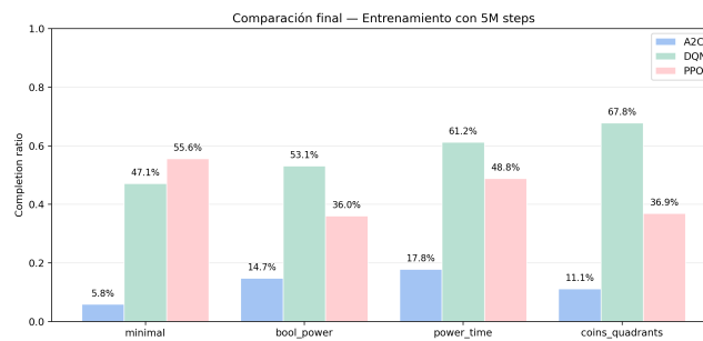
Figura 5.12: Comparativa de completion ratio entre algoritmos con 5M de steps
