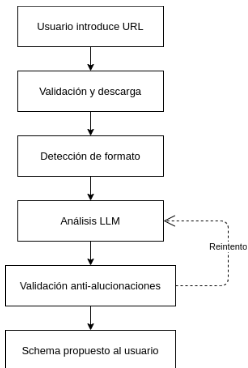
Figura 4.3: Flujo de ingestión y análisis: de URL a schema
