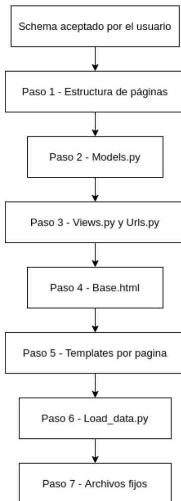
Figura 4.4: Los 7 pasos del generador de proyectos Django
