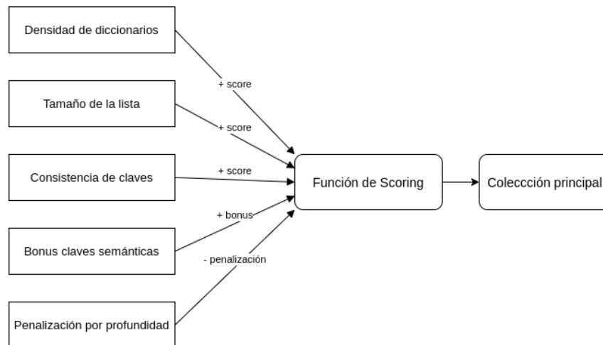
Figura 4.5: Sistema de scoring para la detección de la colección principal
