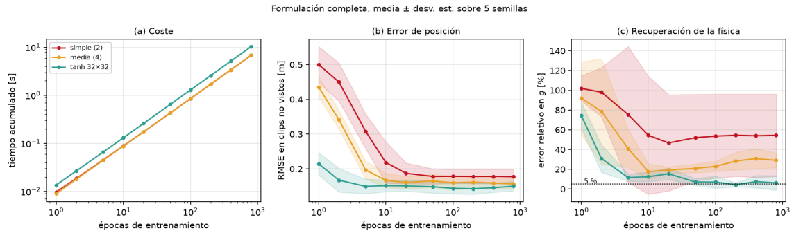
Figura 7: (a) Tiempo acumulado de entrenamiento, estrictamente lineal en el número de épocas. (b) RMSE sobre clips no vistos. (c) Error relativo en la g recuperada. Las líneas muestran la media de las cinco semillas, y la zona sombreada de cada color va desde una desviación estándar por debajo hasta una por encima de esa media; mientras más ancha es, más cambia el resultado de una semilla a otra. Nótese que el eje de épocas es logarítmico: los tramos finales de las curvas cuestan la mayor parte del tiempo total.
