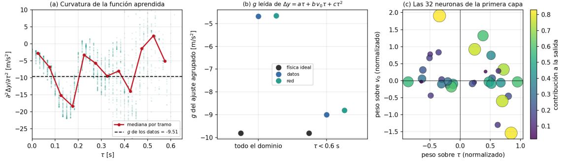
Figura 8: (a) Segunda derivada de la función aprendida, punto a punto sobre los datos de prueba, con su mediana por tramos. Oscila alrededor del valor experimental (línea discontinua) en vez de ser constante. La sombra verde azulado está formada por los valores de la segunda derivada en cada punto de prueba, dibujados semitransparentes; se ordena en columnas porque \tau solo toma los instantes de muestreo del video, separados por 1/60 s. (b) g obtenida ajustando el modelo de MRUV agrupado a la salida de la red y, como control, a los datos experimentales mismos: la red sigue a los datos, no a la física ideal. (c) Pesos de entrada de las 32 neuronas de la primera capa; el tamaño y el color indican su contribución a la salida.
