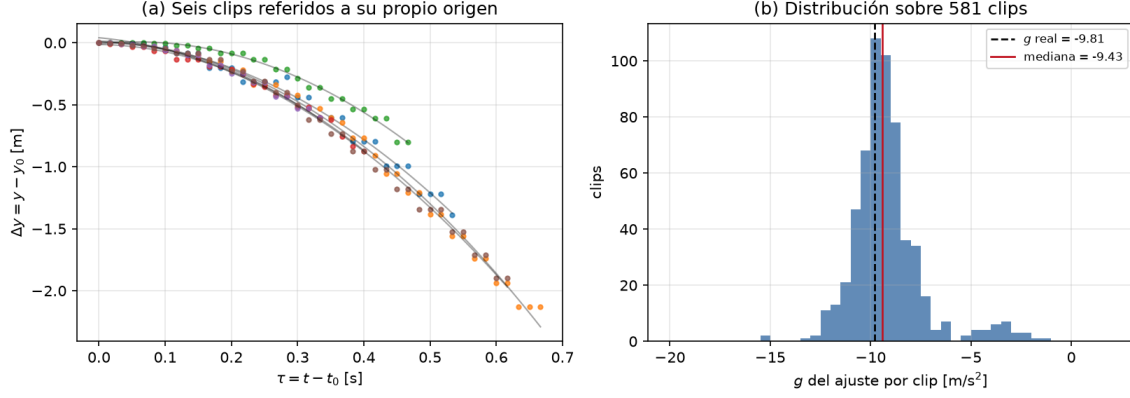
Figura 2: (a) Seis clips experimentales referidos a su propio origen, con su ajuste parabólico. Bajo esta representación todas las trayectorias arrancan en el mismo punto y comparten la misma curvatura, que es lo que fija g . (b) Distribución de la g obtenida ajustando una parábola a cada uno de los 581 clips; la mediana está a un 3.9 % del valor físico.
