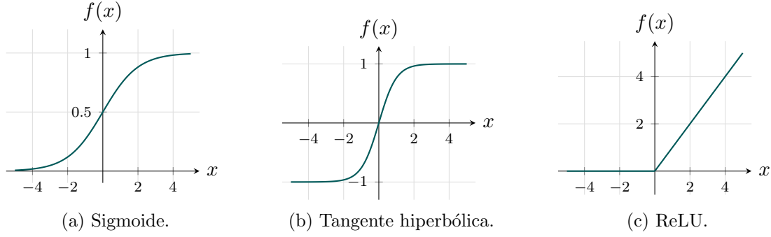
Figura 1: Funciones de activación usadas en este trabajo. Fuente: elaboración propia.
