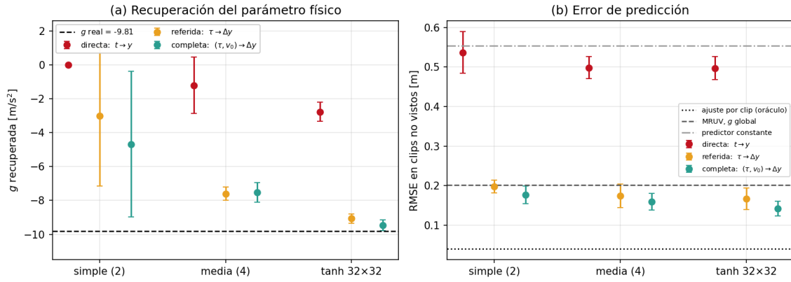
Figura 3: (a) Gravedad recuperada por formulación y arquitectura; la línea discontinua es el valor físico. (b) RMSE sobre clips no vistos, con las tres líneas base como referencia. Barras de error: desviación estándar sobre cinco semillas.
