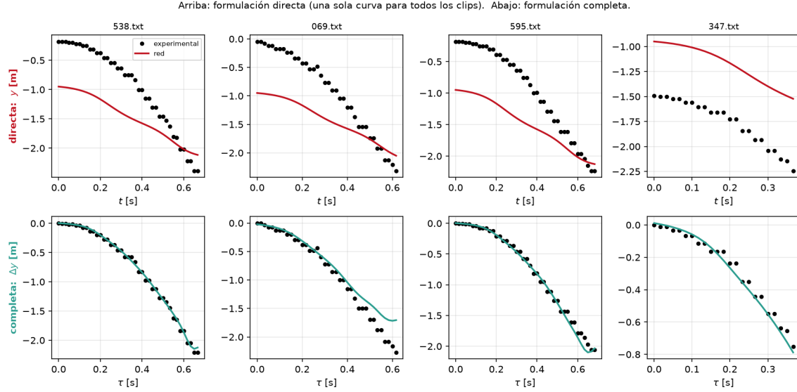
Figura 5: Cuatro clips de prueba con las predicciones de la red \tanh 32 \times 32 . Arriba, formulación directa: la red no puede distinguir un clip de otro y predice esencialmente la misma curva para todos. Abajo, formulación completa: la red reproduce la trayectoria de cada clip.
