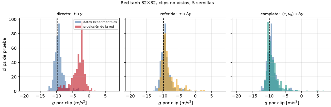
Figura 4: Distribución de la g estimada clip por clip para la red tanh 32 \times 32 ; en azul la de los datos experimentales y en color la de las predicciones. Al pasar de la formulación directa a la completa las dos distribuciones dejan de estar separadas y se superponen.
