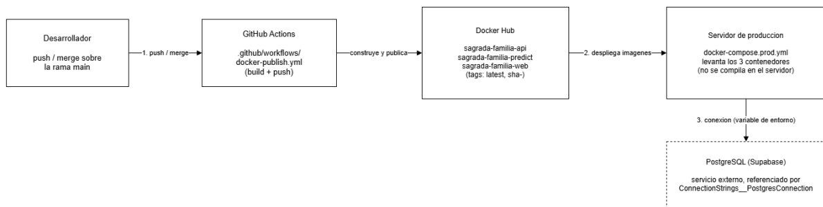
Figura 3. Flujo de integración y despliegue continuo.
