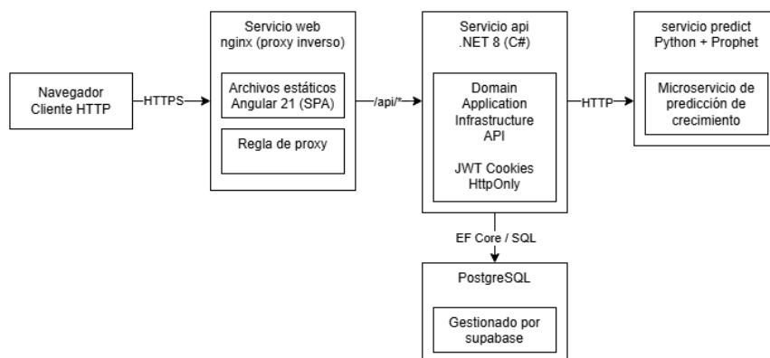
Figura 1. Arquitectura general del sistema.
