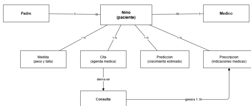
Figura 2. Relaciones centrales del modelo de dominio.
