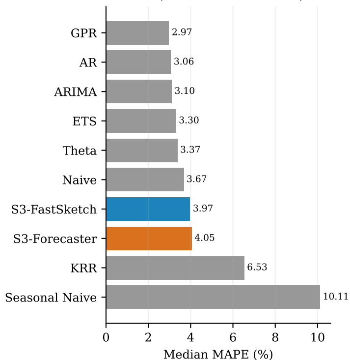
M4 (available models: 10)
