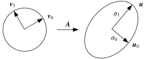
Slika 2.5: Geometrijsko tumačenje SVD/PCA transformacije. Preuzeto iz [1], Slika A.1, str. 738.
