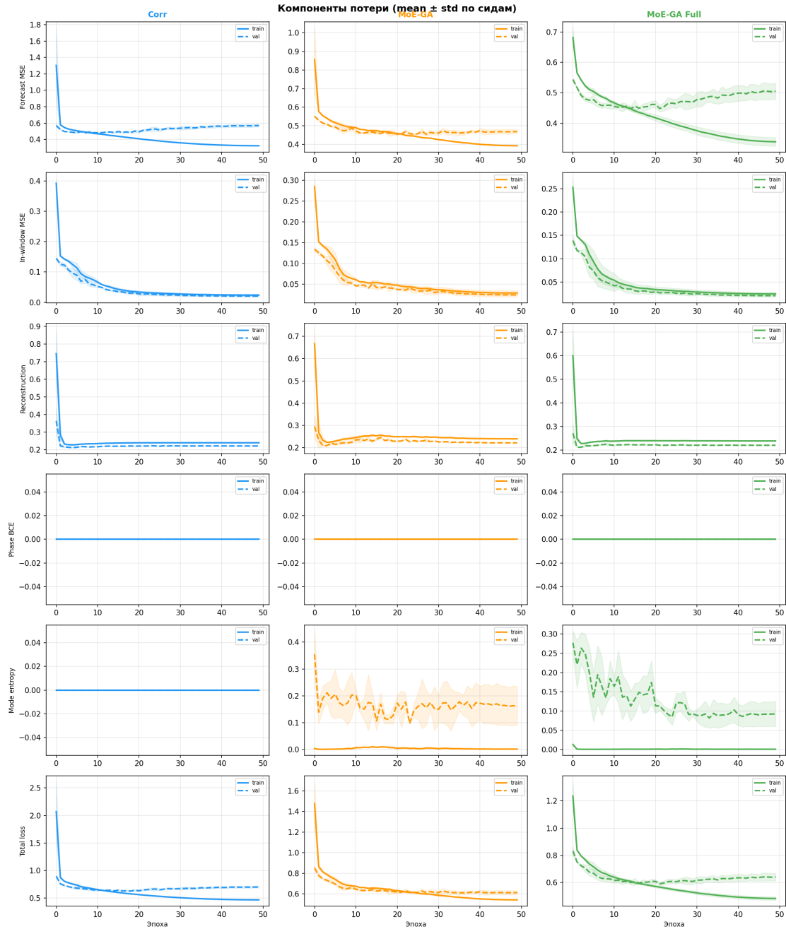
Рис. 10. ЭЭГ: компоненты функционала потерь по эпохам обучения. Phase BCE тождественно равна нулю: метка режима в ЭЭГ-экспериментах не подавалась (раздел 5.4).
