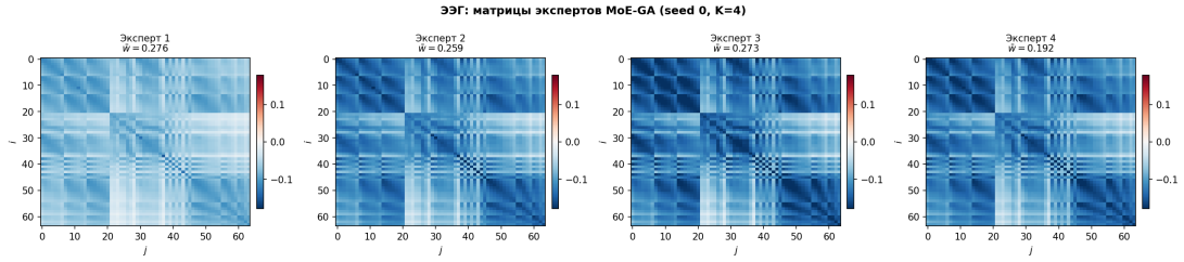
Рис. 16. ЭЭГ: матрицы экспертов MoE-GA ( K = 4 ). Средние веса: \bar{w} \approx [0,28, 0,26, 0,27, 0,19] . Равномерное использование всех четырёх экспертов указывает на отсутствие монополизации и покрытие разных паттернов связности.
