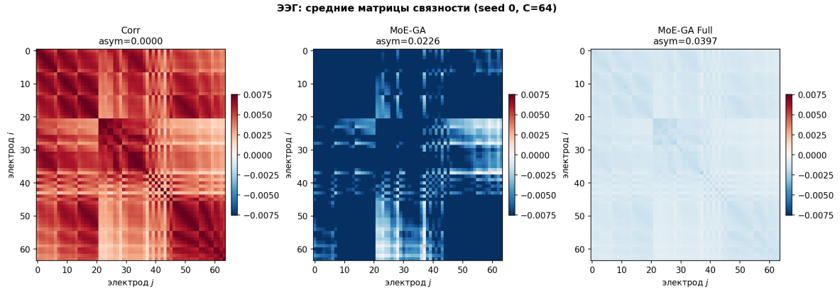
Рис. 15. ЭЭГ: средние матрицы \hat{A} по всем сэмплам ( C = 64 ): Corr (слева), MoE-GA (центр), MoE-GA Full (справа). Мера асимметрии: 0, 0,023, 0,040 соответственно. Видна блочная структура, соответствующая анатомическим группам электродов.
