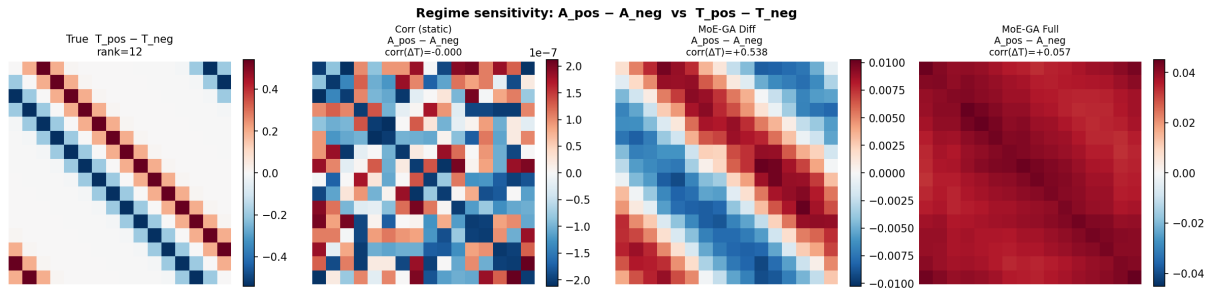
Рис. 13. Drift-ring: разности \hat{A}_+ - \hat{A}_- (чувствительность к смене режима). У Corr разность близка к нулю; у MoE-GA — выражена.
