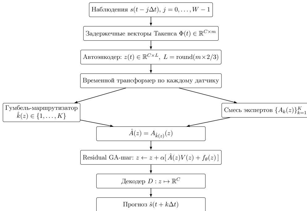
Рис. 1. Схема модели MoE-GA. Состояние сжимается до латента z(t) размерности L = \text{round}(m \times 2/3) ; жёсткий маршрутизатор Гумбеля выбирает ровно одного эксперта из смеси K компонент; выбранное ядро даёт асимметричный оператор \hat{A}(z) , по которому далее выполняется один residual-шаг graph attention. В варианте MoE-GA Full дополнительно присутствует реакционный член f_\theta(z) .
