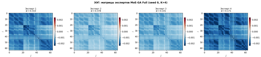
Рис. 17. ЭЭГ: матрицы экспертов MoE-GA Full ( K = 4 ). Средние веса: \bar{w} \approx [0,31, 0,38, 0,14, 0,17] . Эксперт 2 доминирует — кодирует низкочастотную ( \delta ) компоненту; остальные специализированы на более локальных связях.
