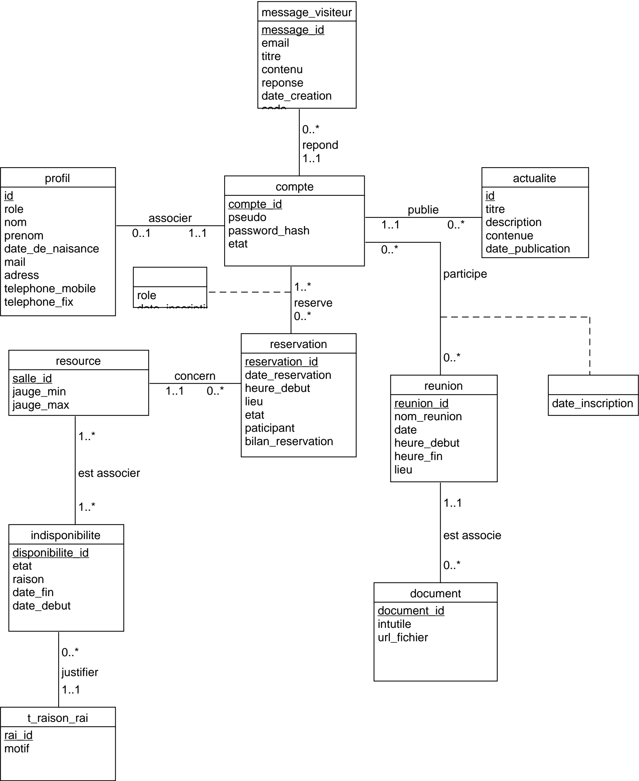
Diagram UML de classe de projet resaweb "LAN party"
