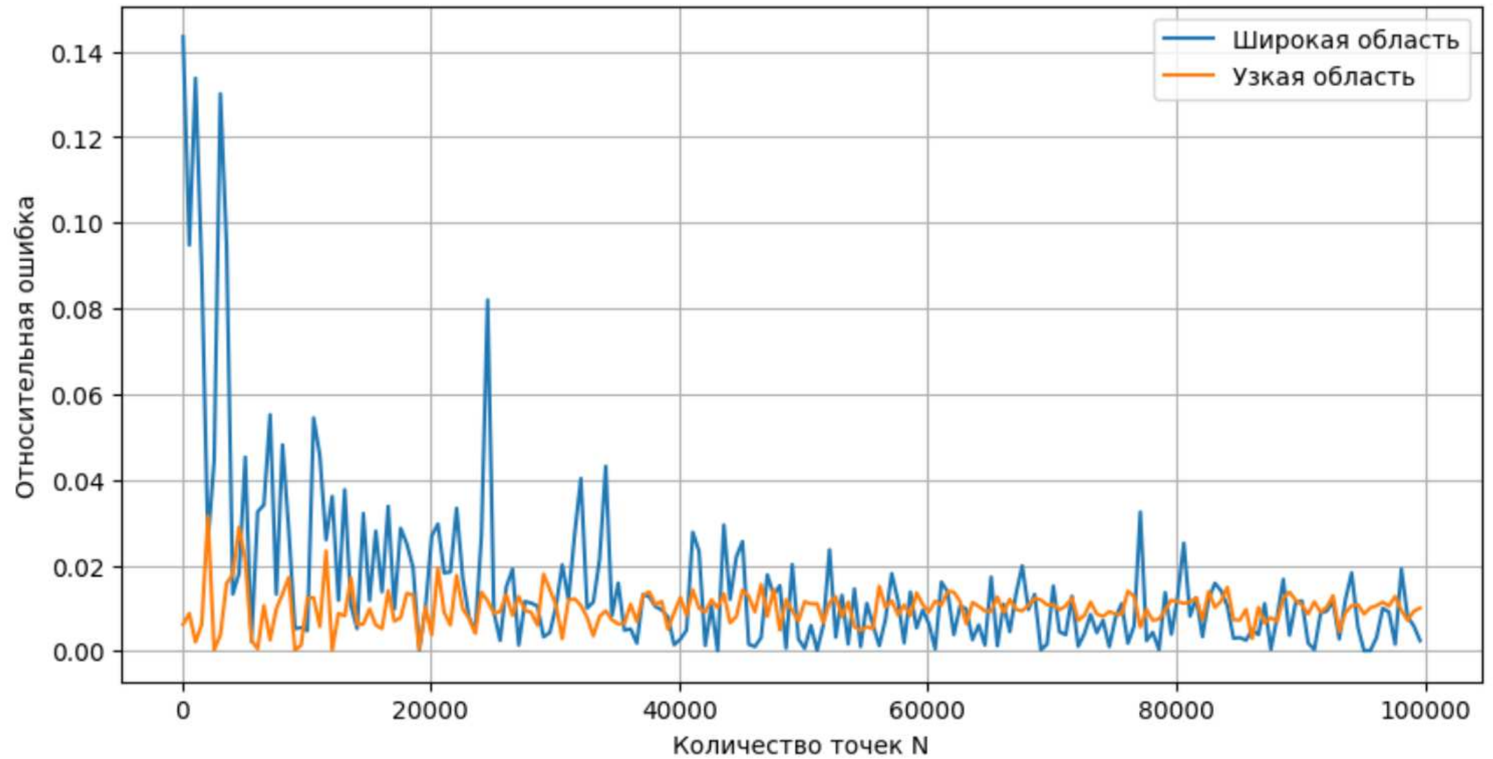
Относительная ошибка vs N
