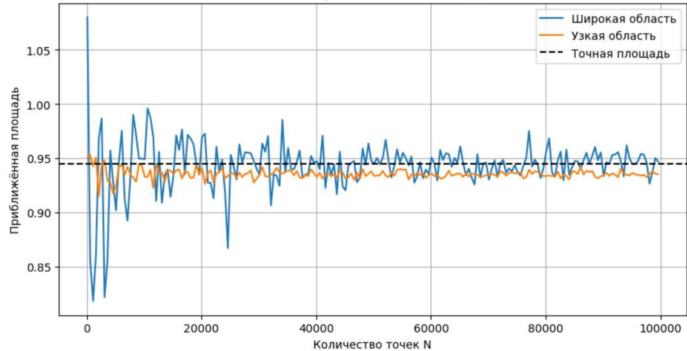
Зависимость приближённой площади от N
