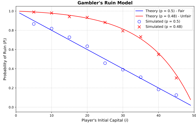
Rysunek 3: Prawdopodobieństwo ruiny gracza w zależności od kapitału początkowego z N = 50 .
