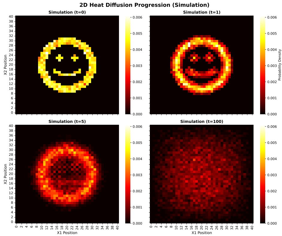
Rysunek 6: Symulacja ewolucji systemu dla bardziej skomplikowanych warunków początkowych.
