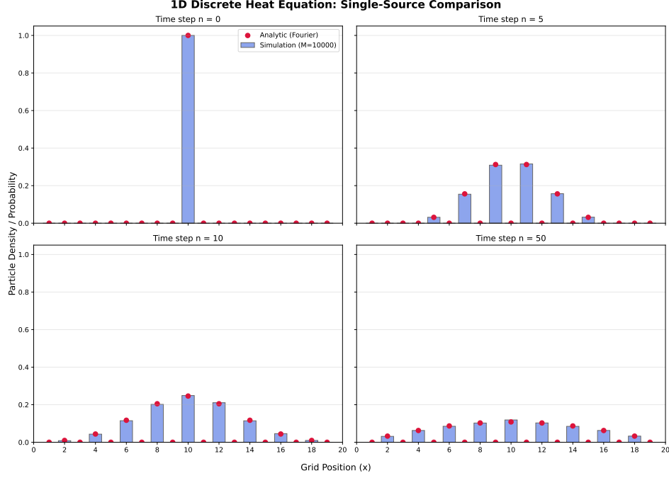
Rysunek 4: Ewolucja układu z jednym źródłem.
