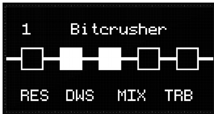
Fig. 4.39 - Interfaccia grafica
