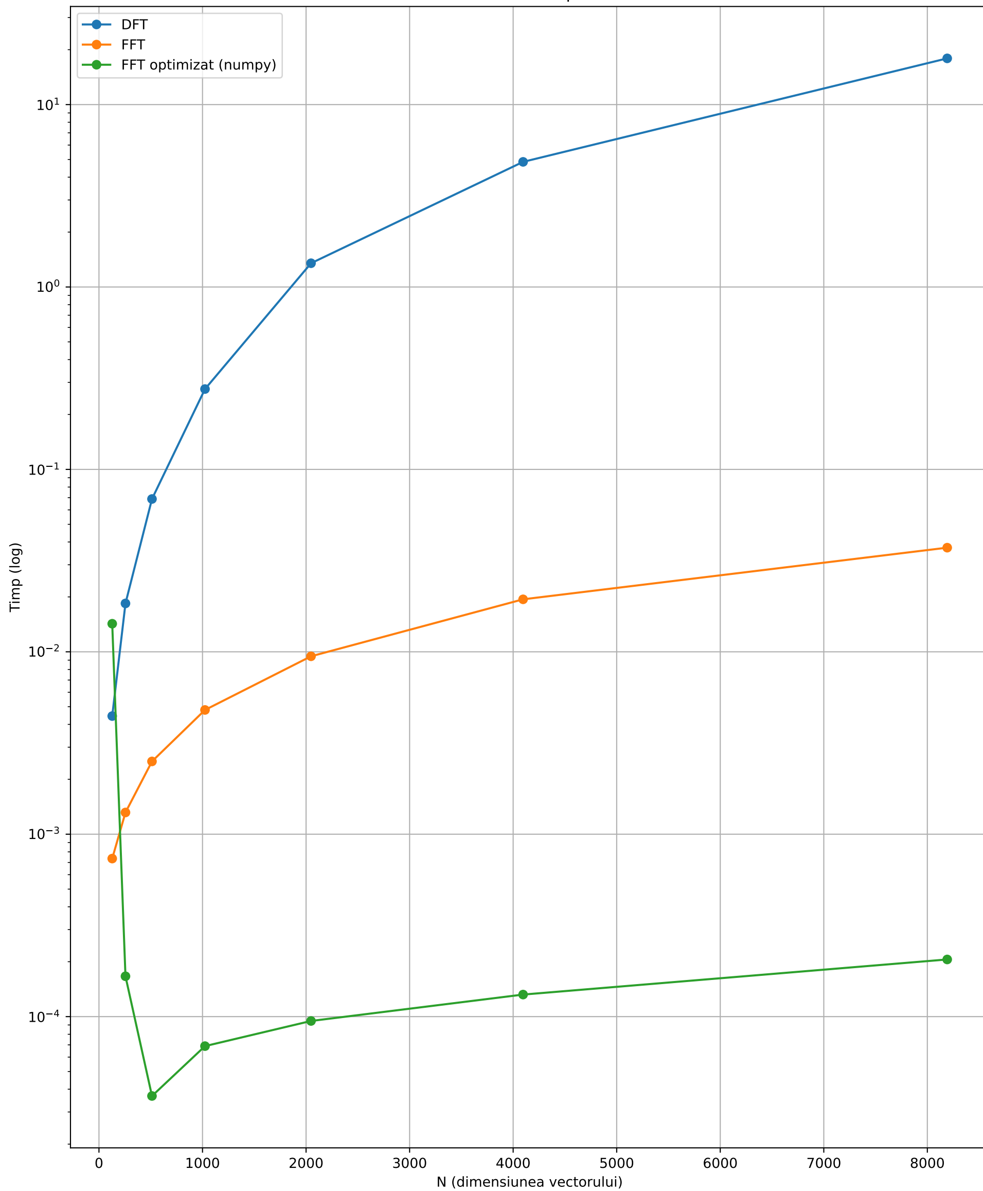
DFT vs FFT vs np.fft.fft
