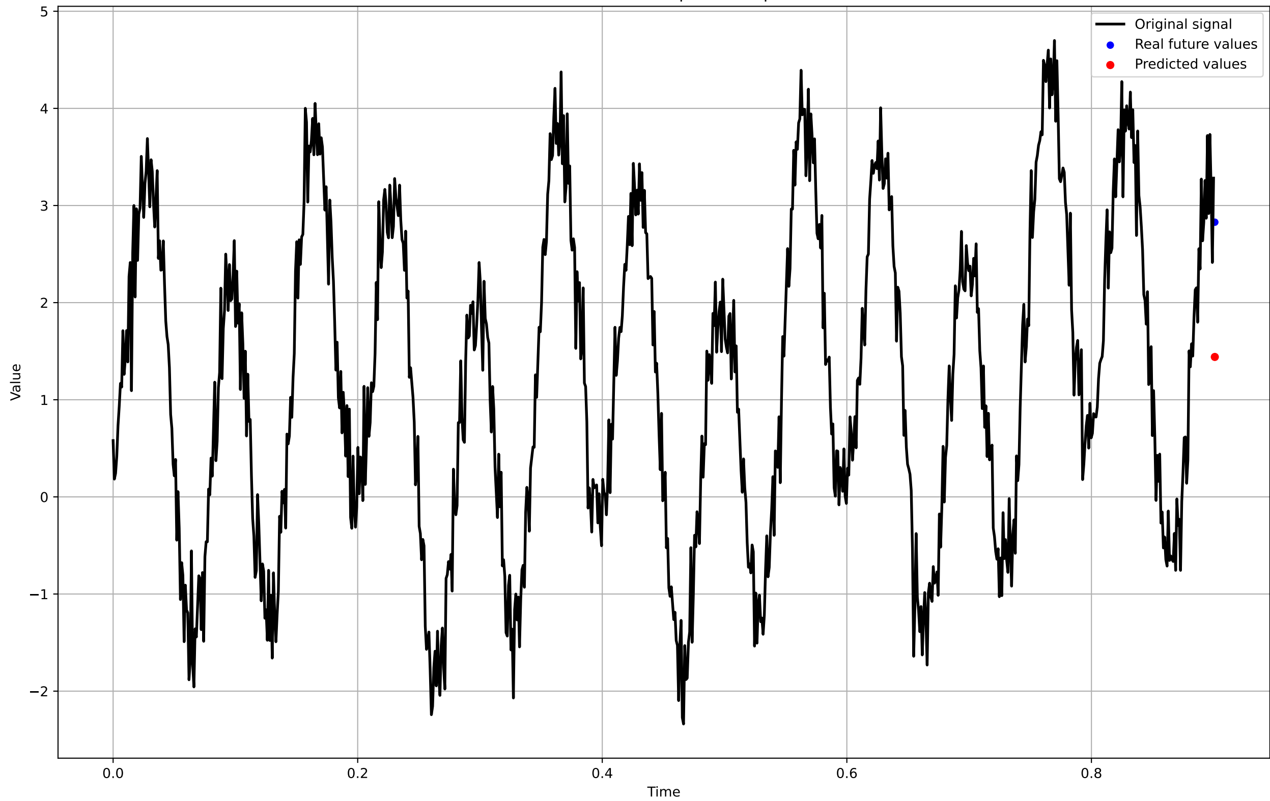
Predictie ARMA cu p = 15 si q = 9
